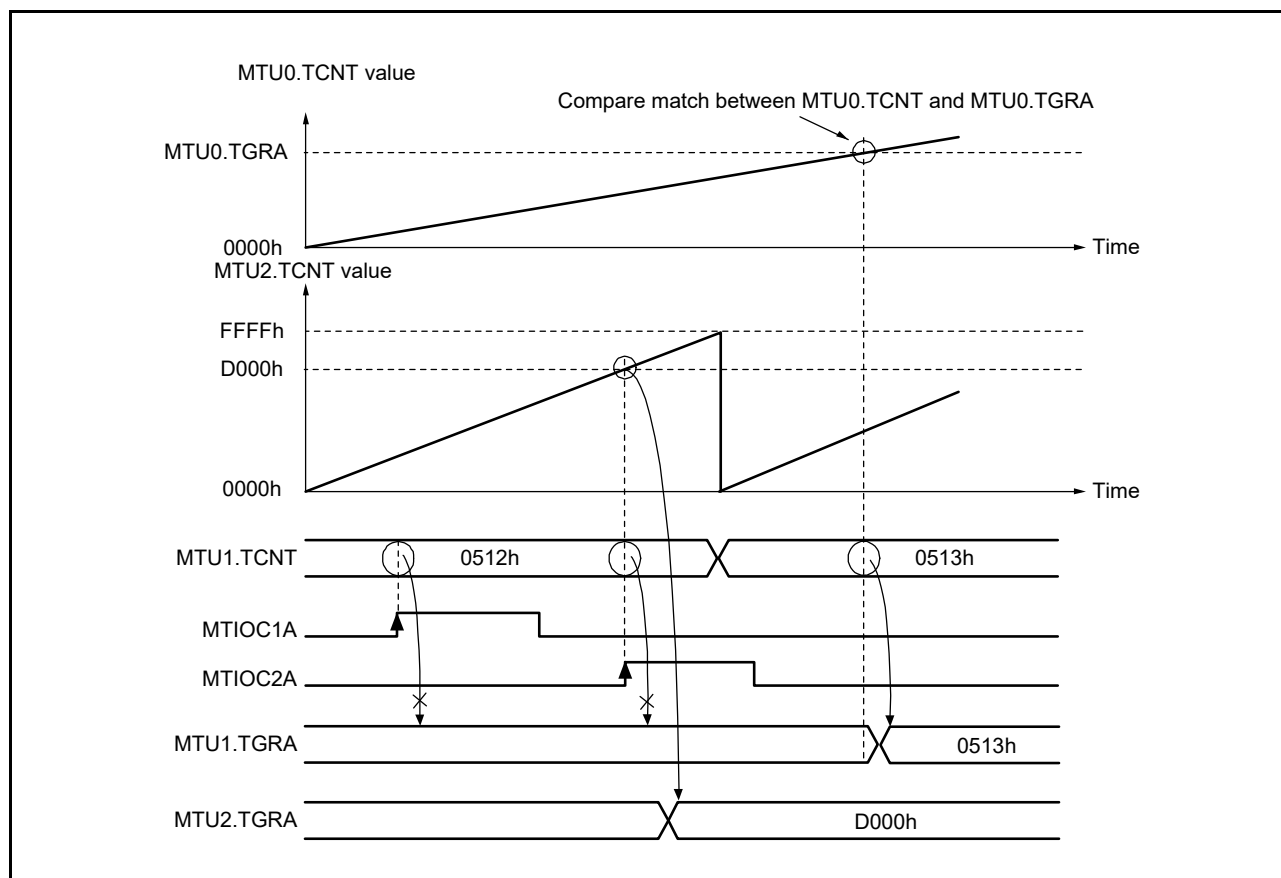
Figure 20.25 Cascaded Operation Example (d)
