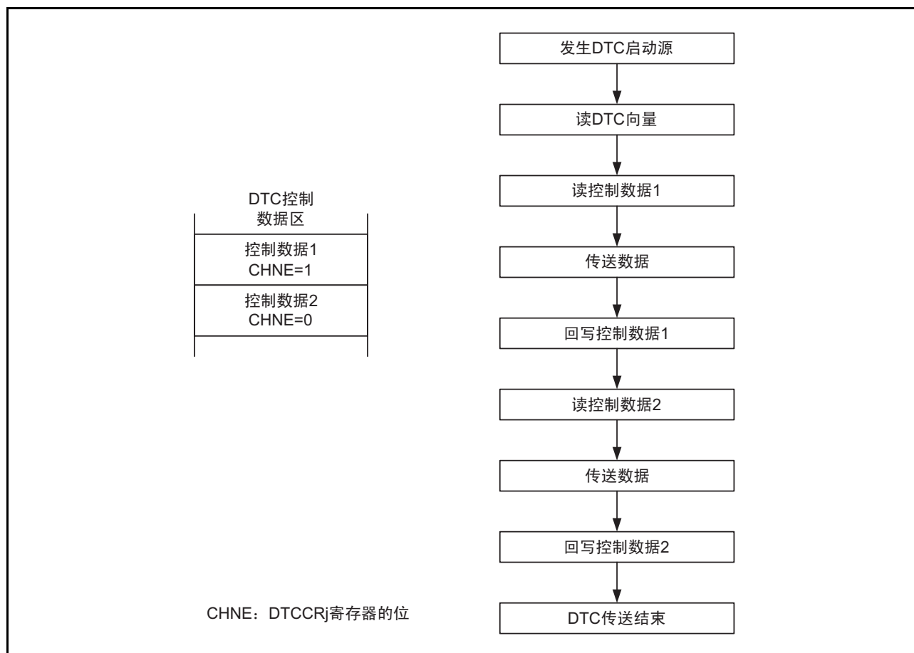
图 15.10 链传送的流程图
