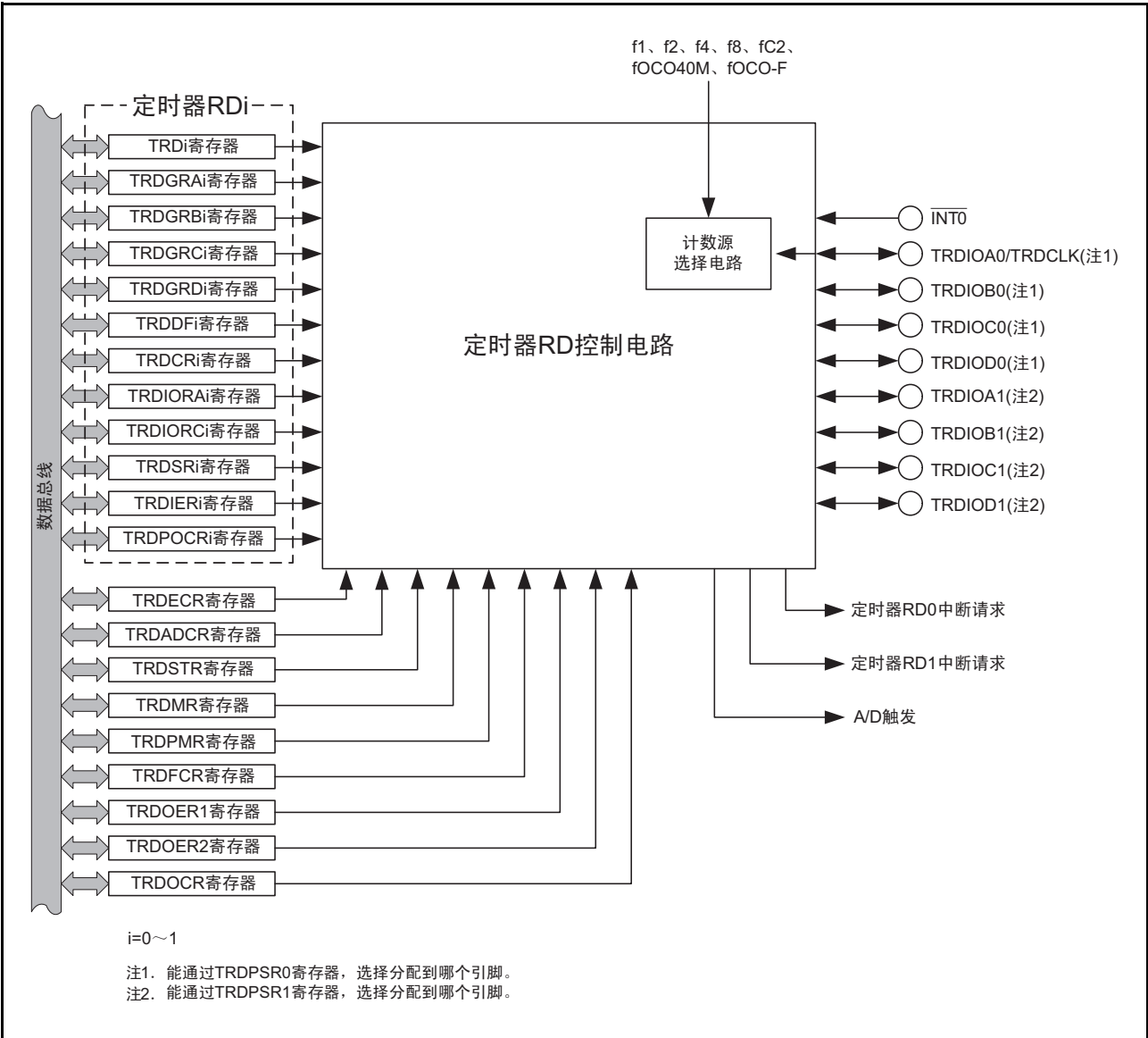
图 20.1 定时器 RD 的框图
