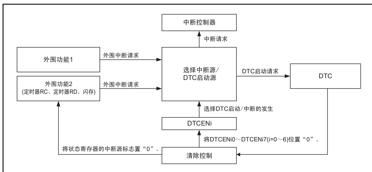
图 15.2 DTC 启动源的控制框图
