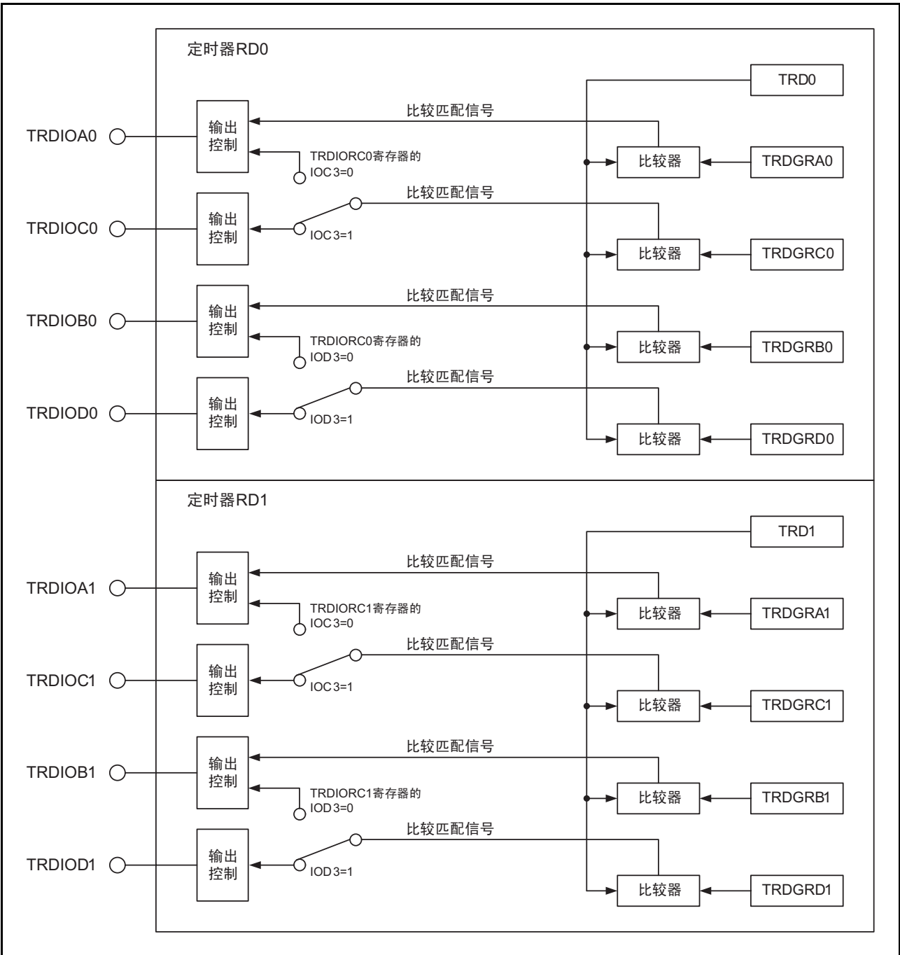
图 20.10 输出比较功能的框图
