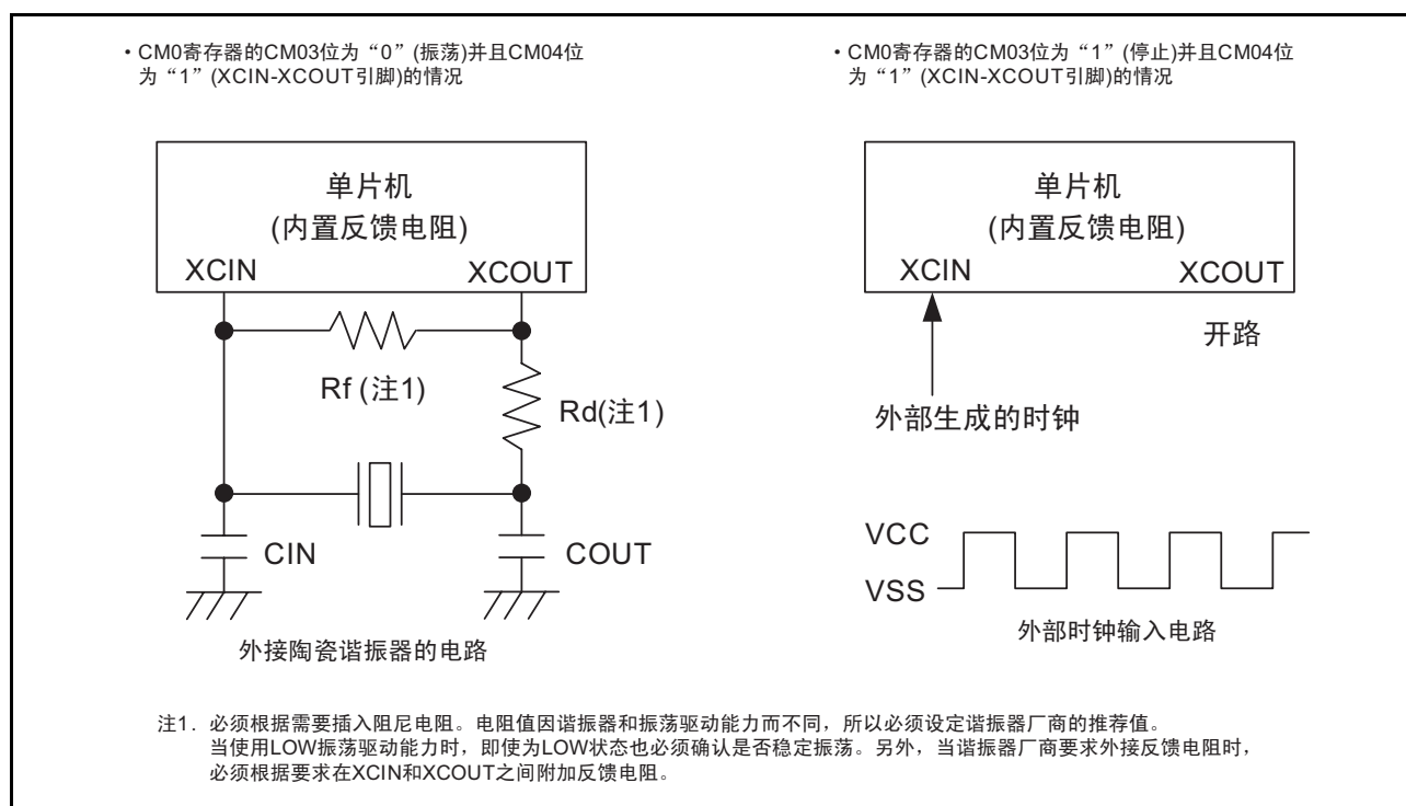
图 9.5 XCIN 时钟的连接电路例子
