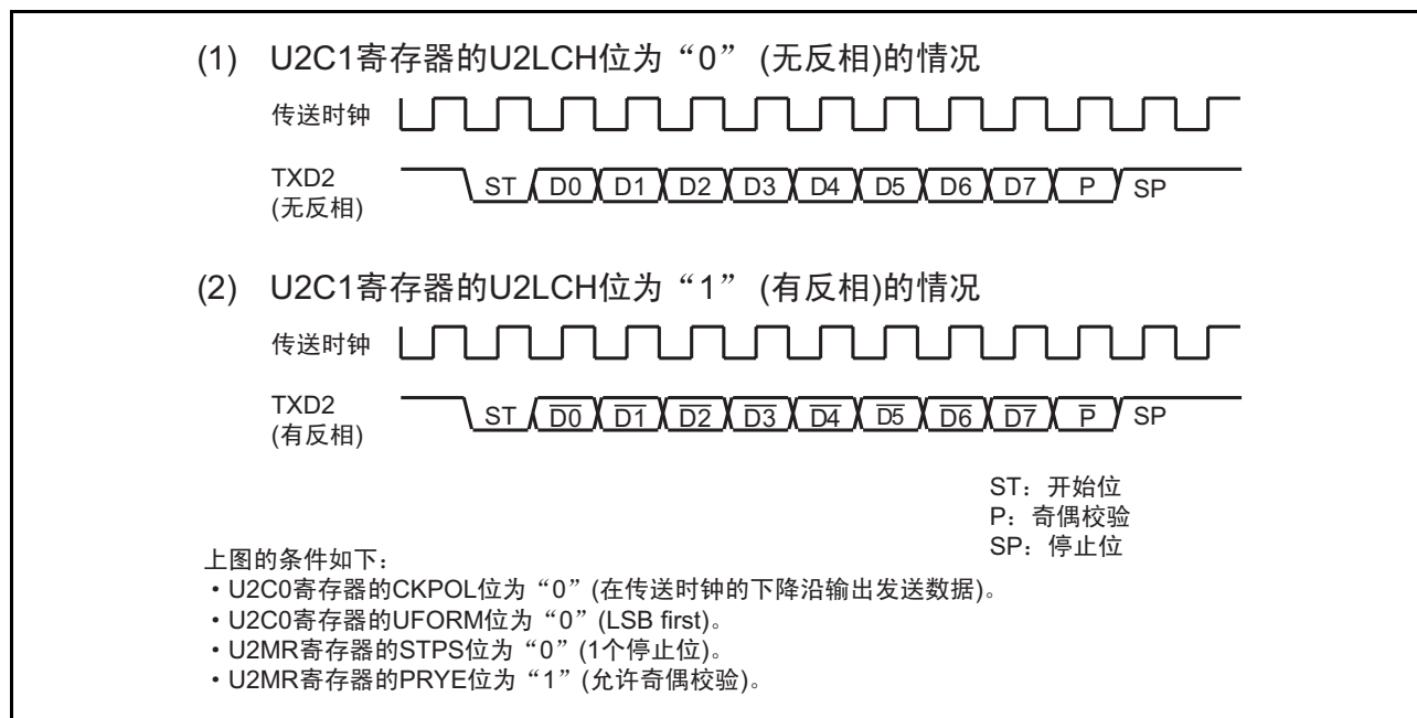
图 23.10 串行数据的逻辑
