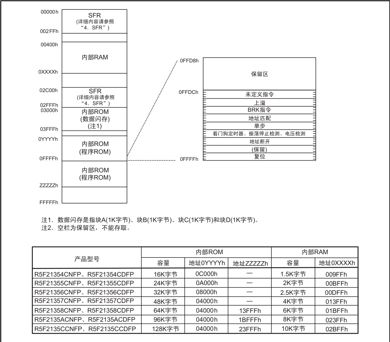
图 3.1 R8C/35C 群的存储器分配图
