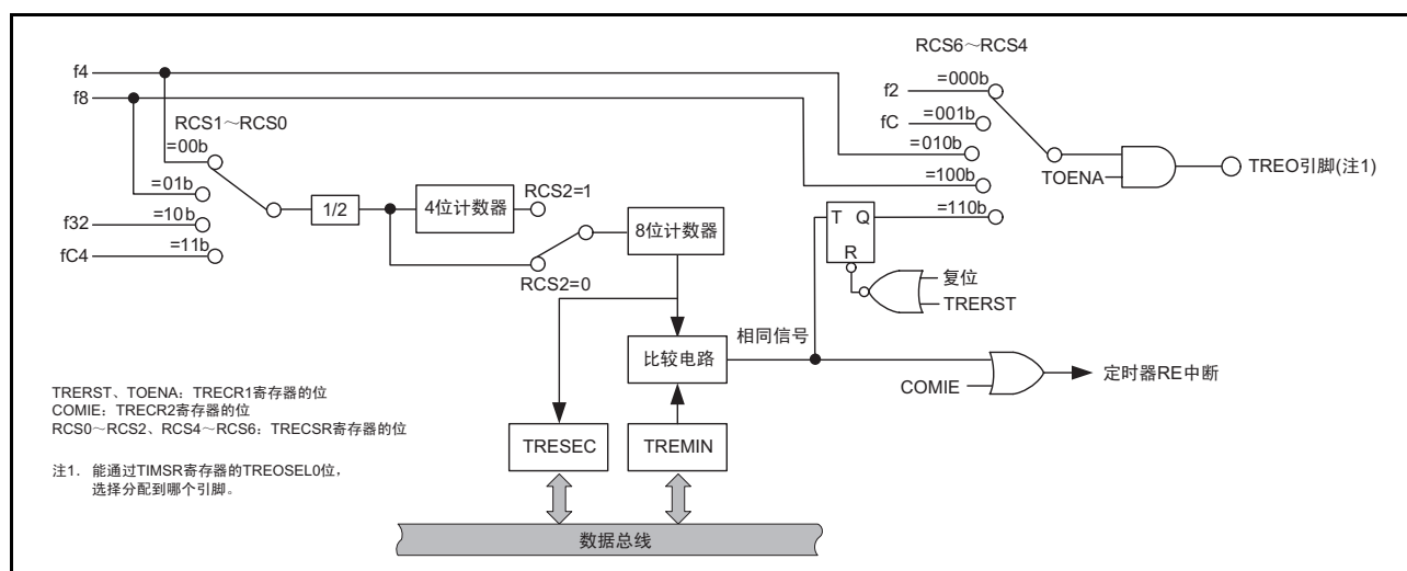
图 21.4 输出比较模式的框图
