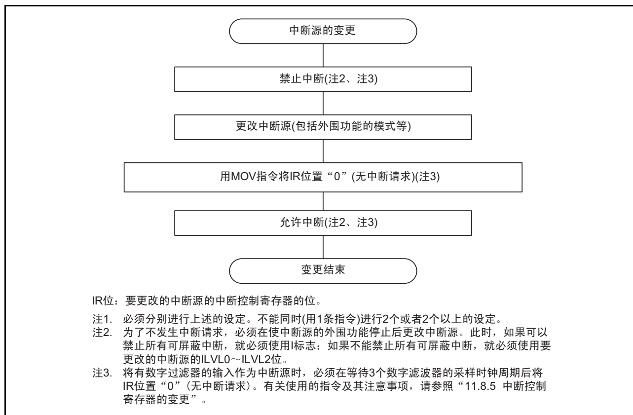
图 11.13 中断源的变更步骤例子
