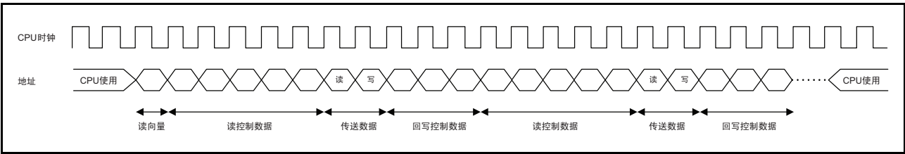
图 15.12 链传送时的 DTC 的运行时序例子
