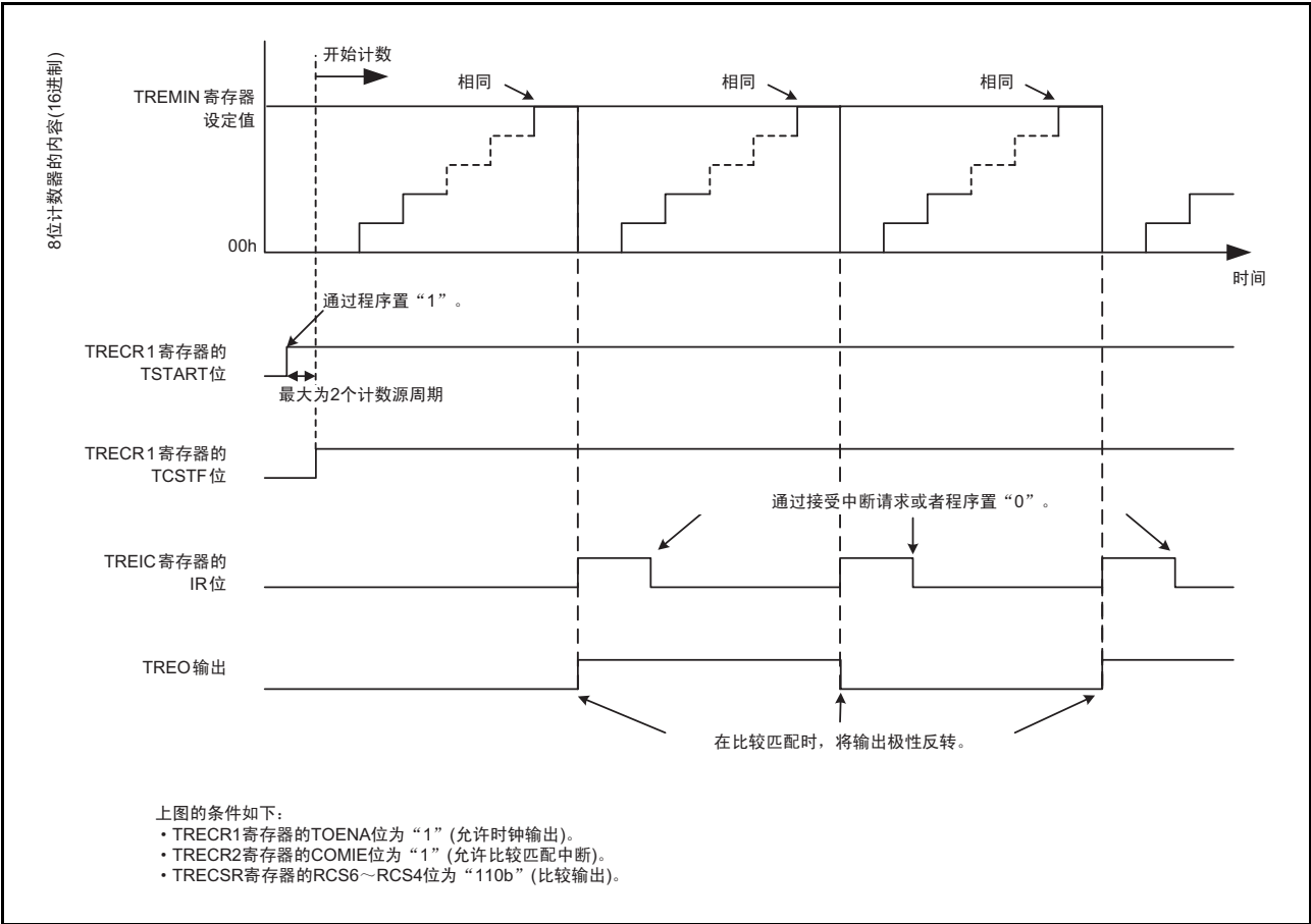
图 21.5 输出比较模式的运行例子
