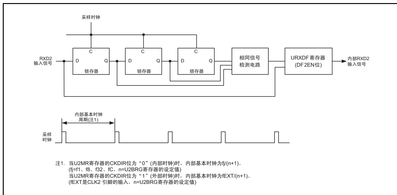
图 23.22 RXD2 数字滤波器电路的框图
