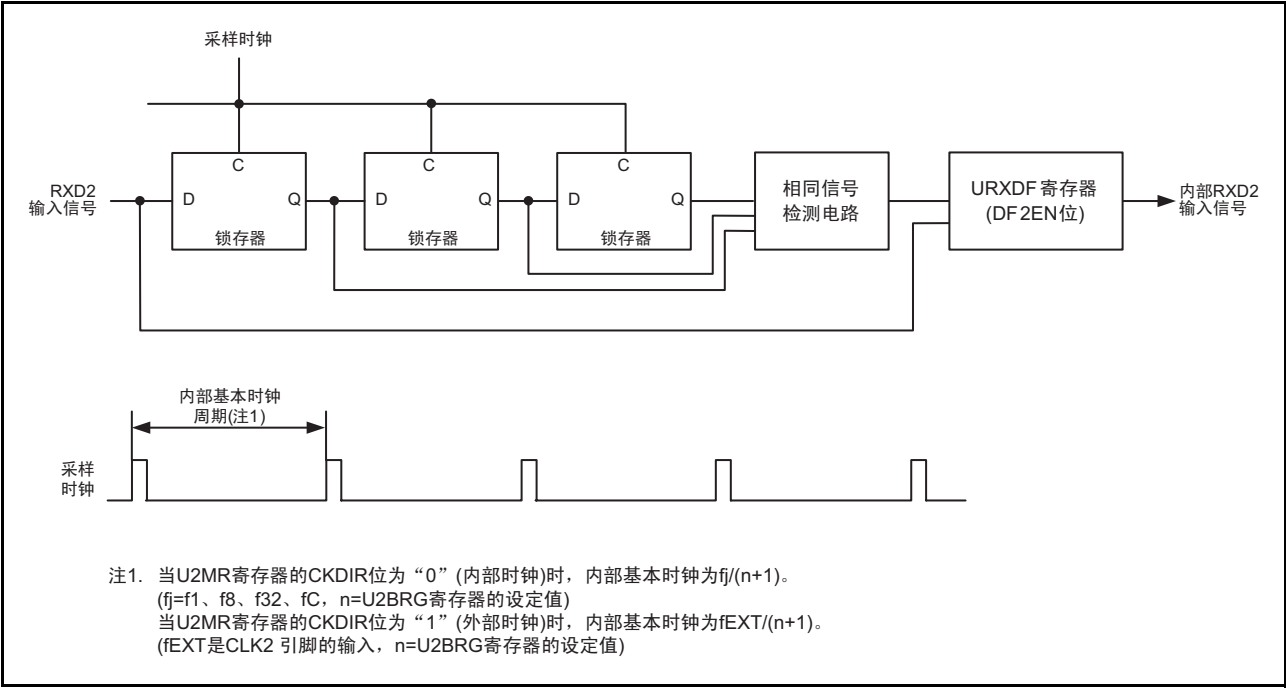
图 23.12 RXD2 数字滤波器电路的框图
