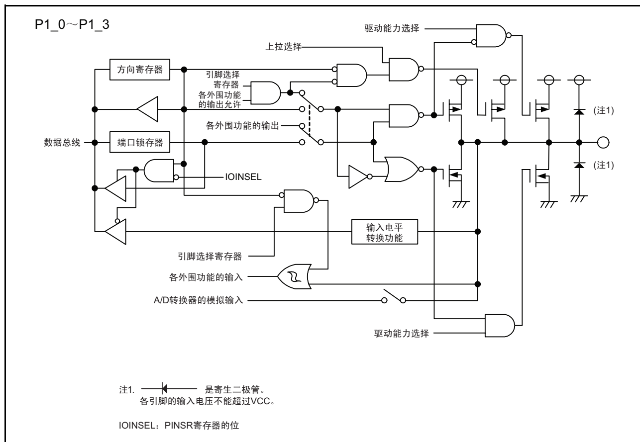
图 7.2 I/O 端口的结构 (2)
