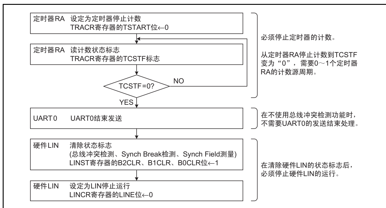
图 27.10 硬件 LIN 通信结束的流程图例子
