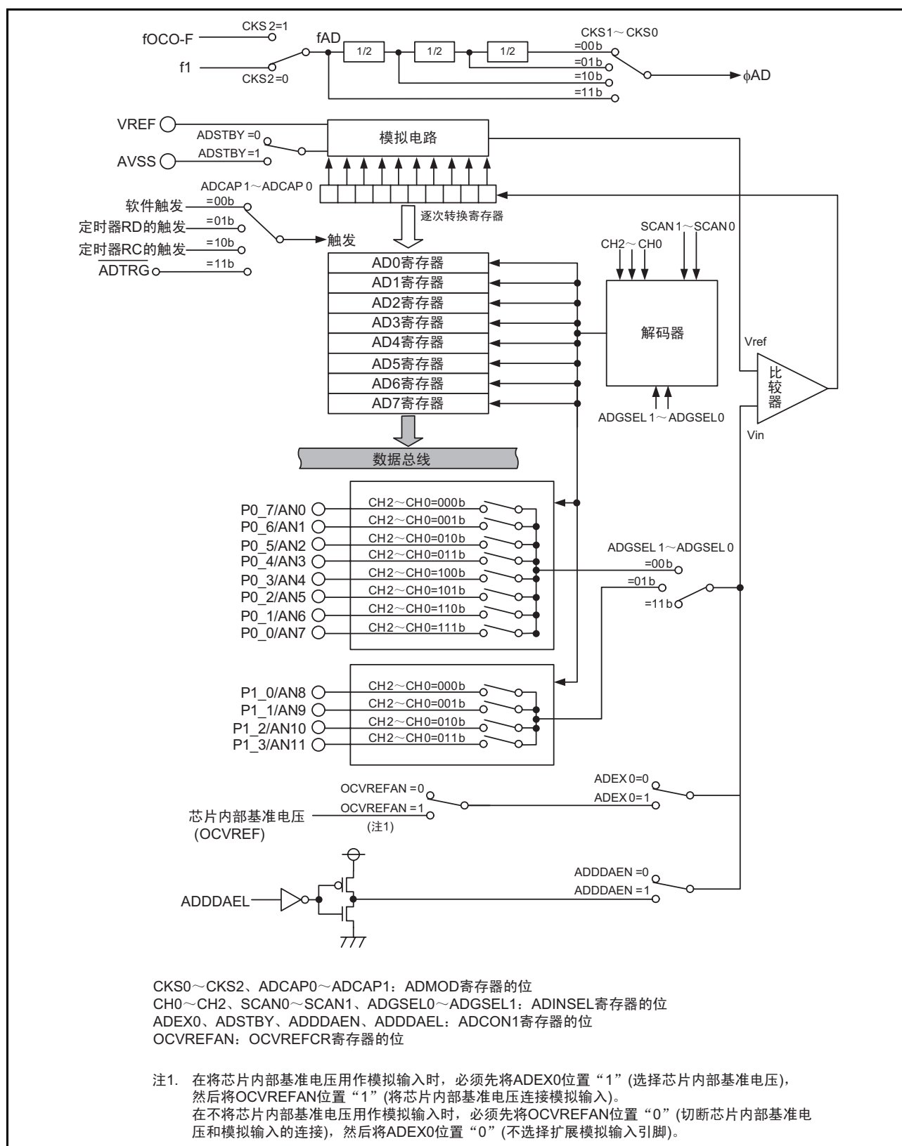
图 28.1 A/D 转换器的框图
