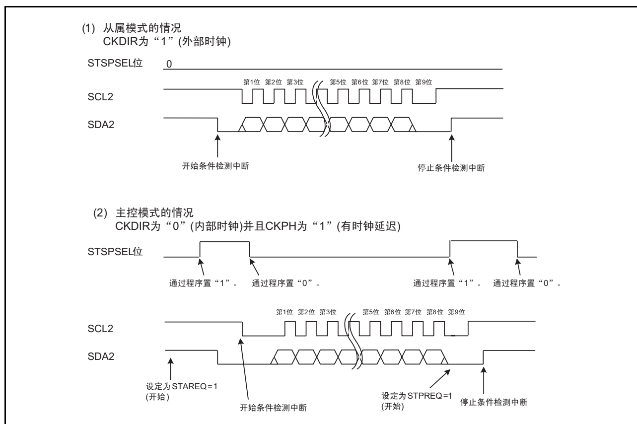
图 23.16 STSPSEL 位的功能
