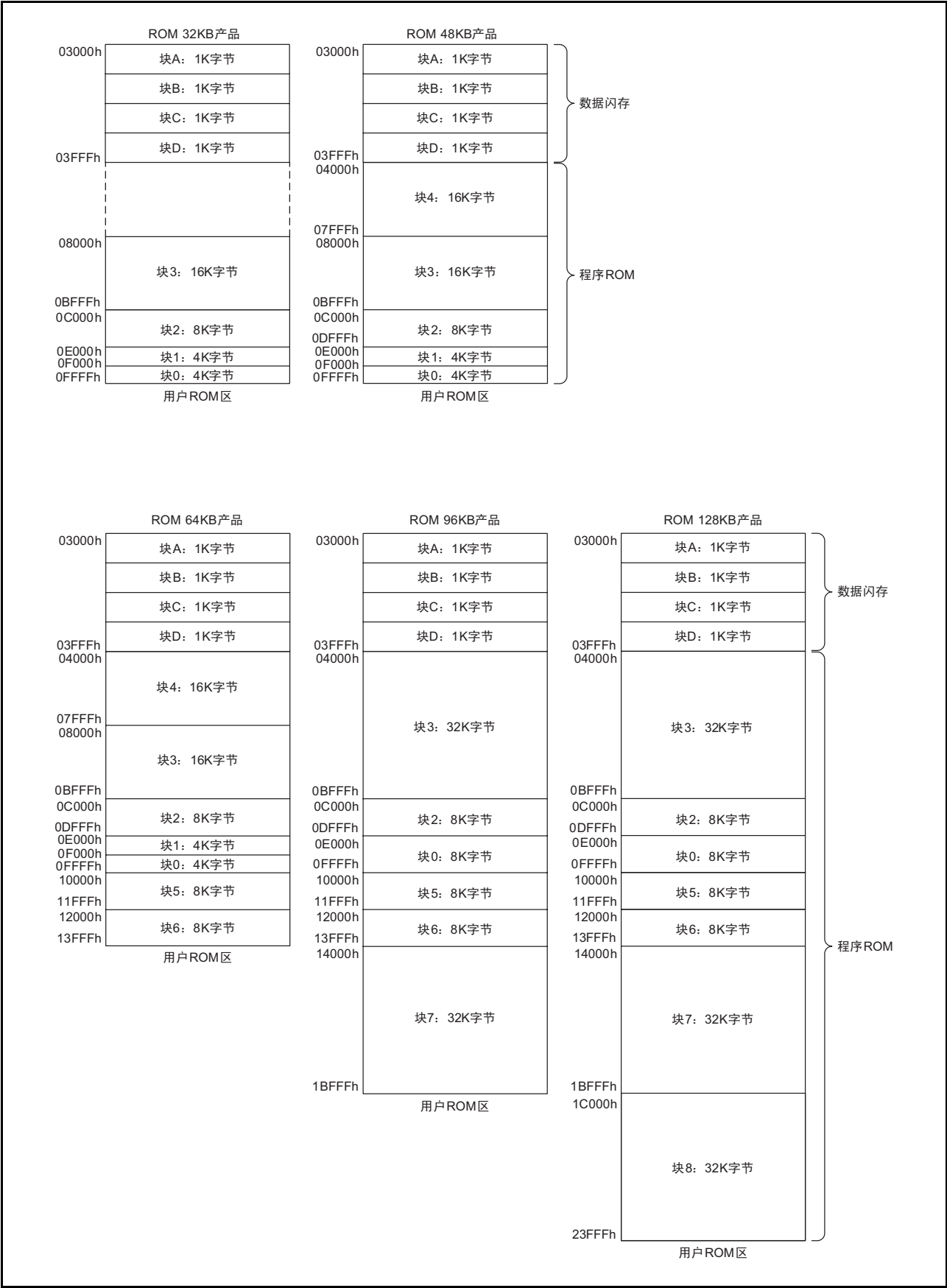
图 31.2 R8C/35C 群的闪存框图 (2)
