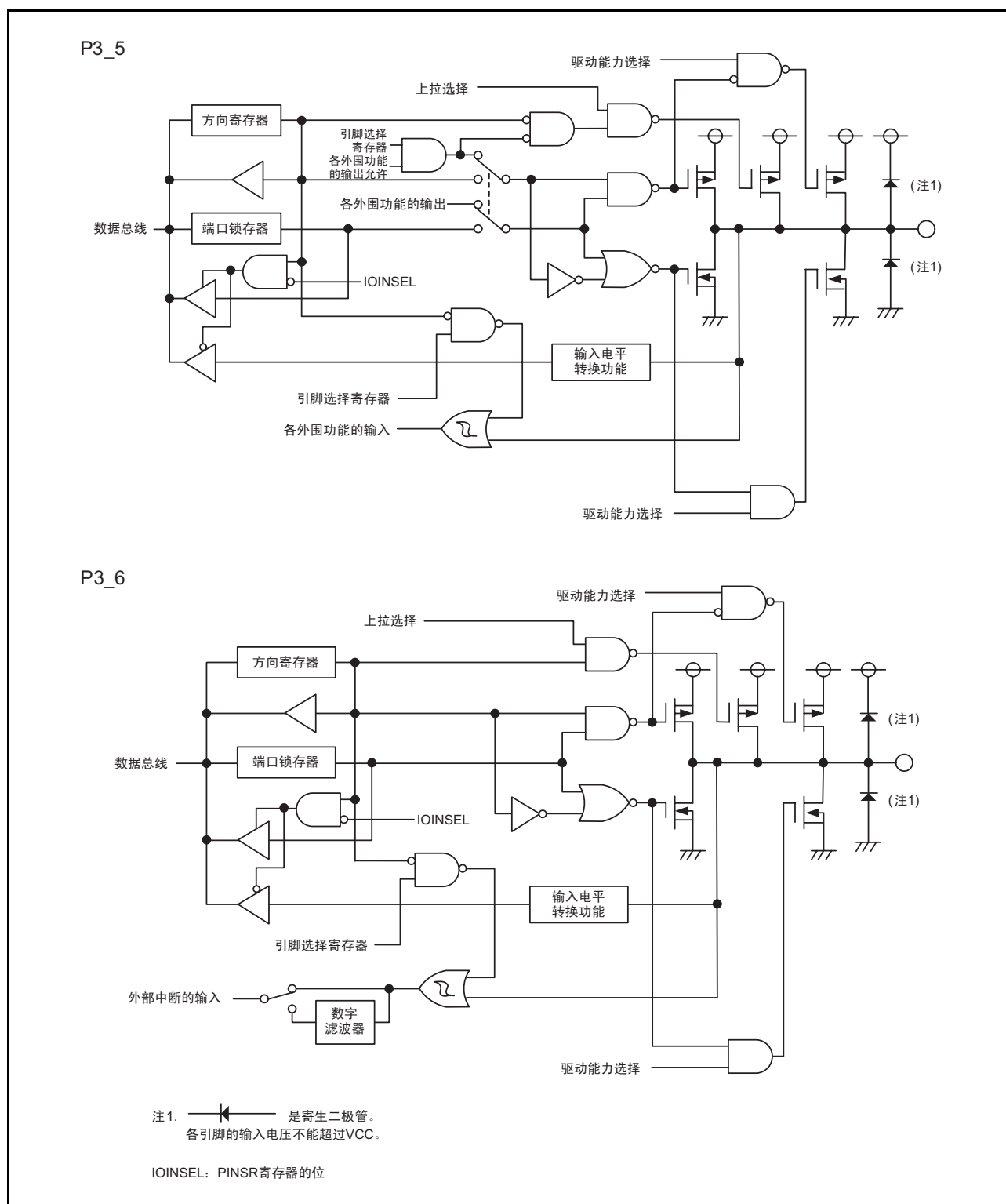
图 7.8 I/O 端口的结构 (8)
