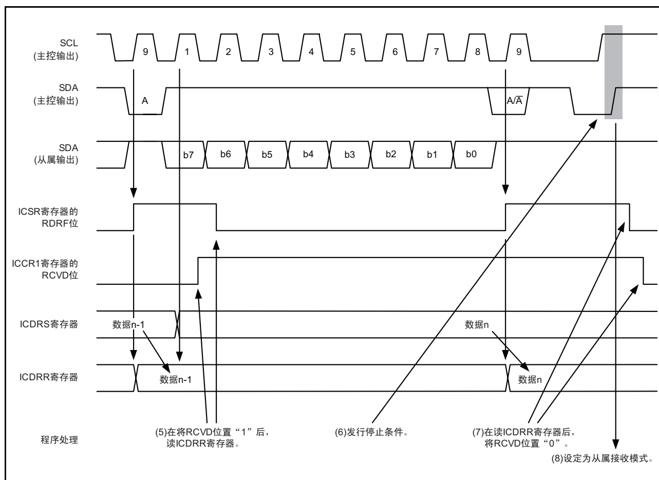
图 26.8 主控接收模式的运行时序 (I 2 C 总线接口模式) (2)
