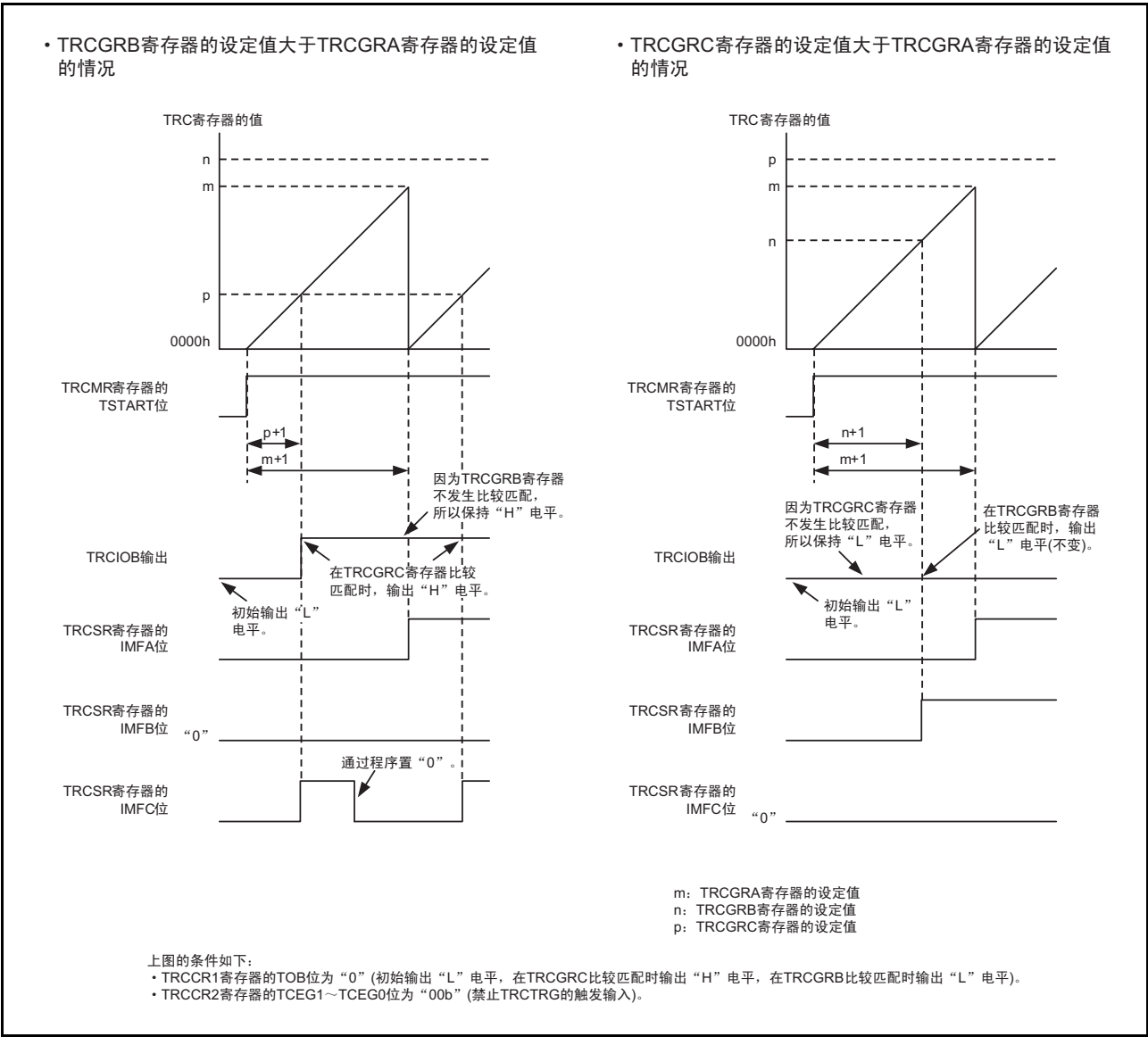
图 19.19 PWM2 模式的运行例子（占空比为 0% 和 100%）
