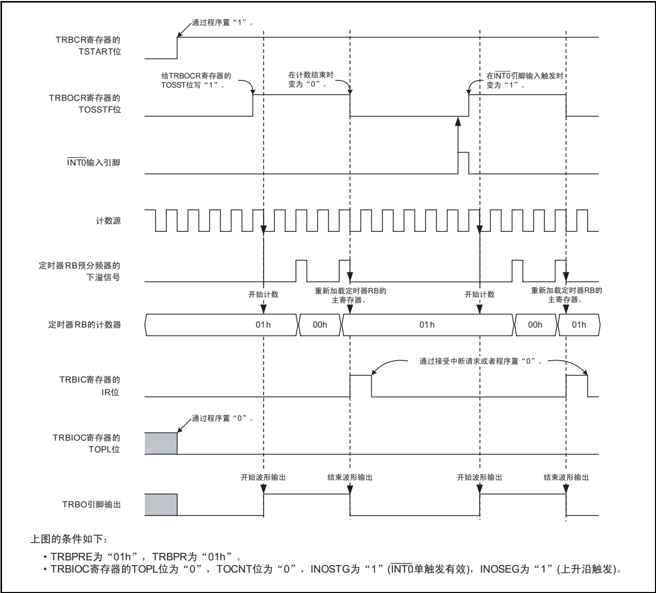
图 18.4 可编程单触发发生模式的运行例子
