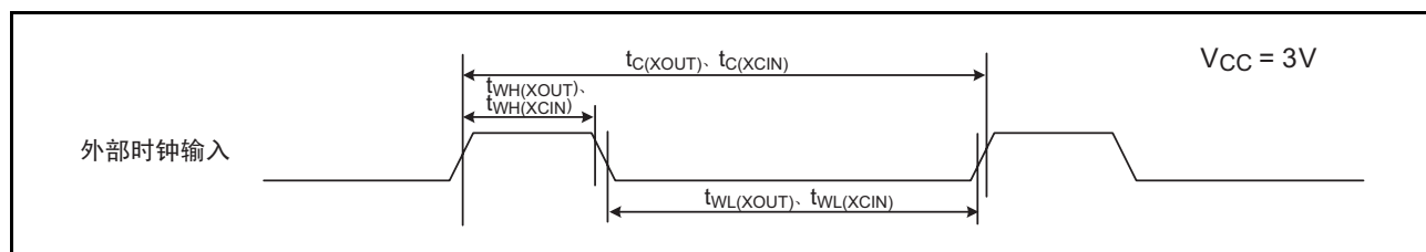
图 33.12 V_{CC}=3V 时的外部时钟输入时序
