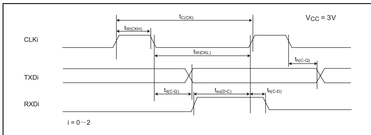
图 33.14 V_{CC}=3V 时的串行接口时序
