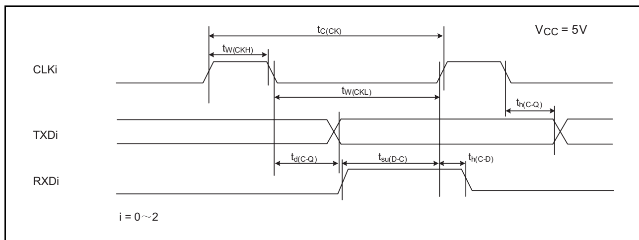
图 33.10 V_{CC}=5V 时的串行接口时序
