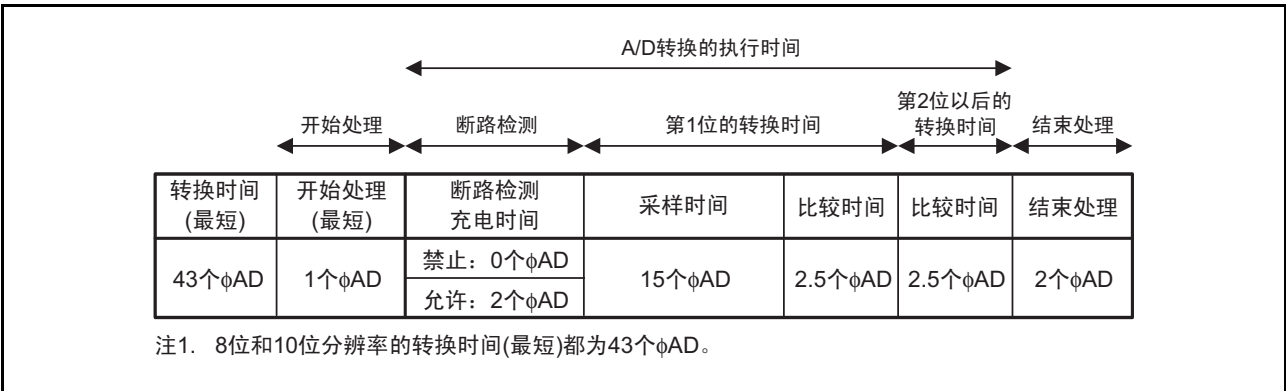
图 28.3 A/D 转换周期数 ( \phi_{AD}=f_{AD} )
