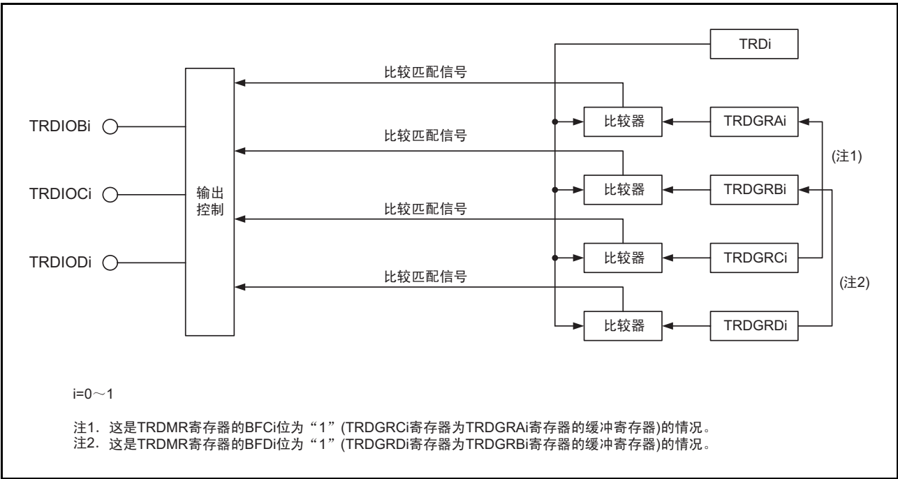
图 20.14 PWM 模式的框图
