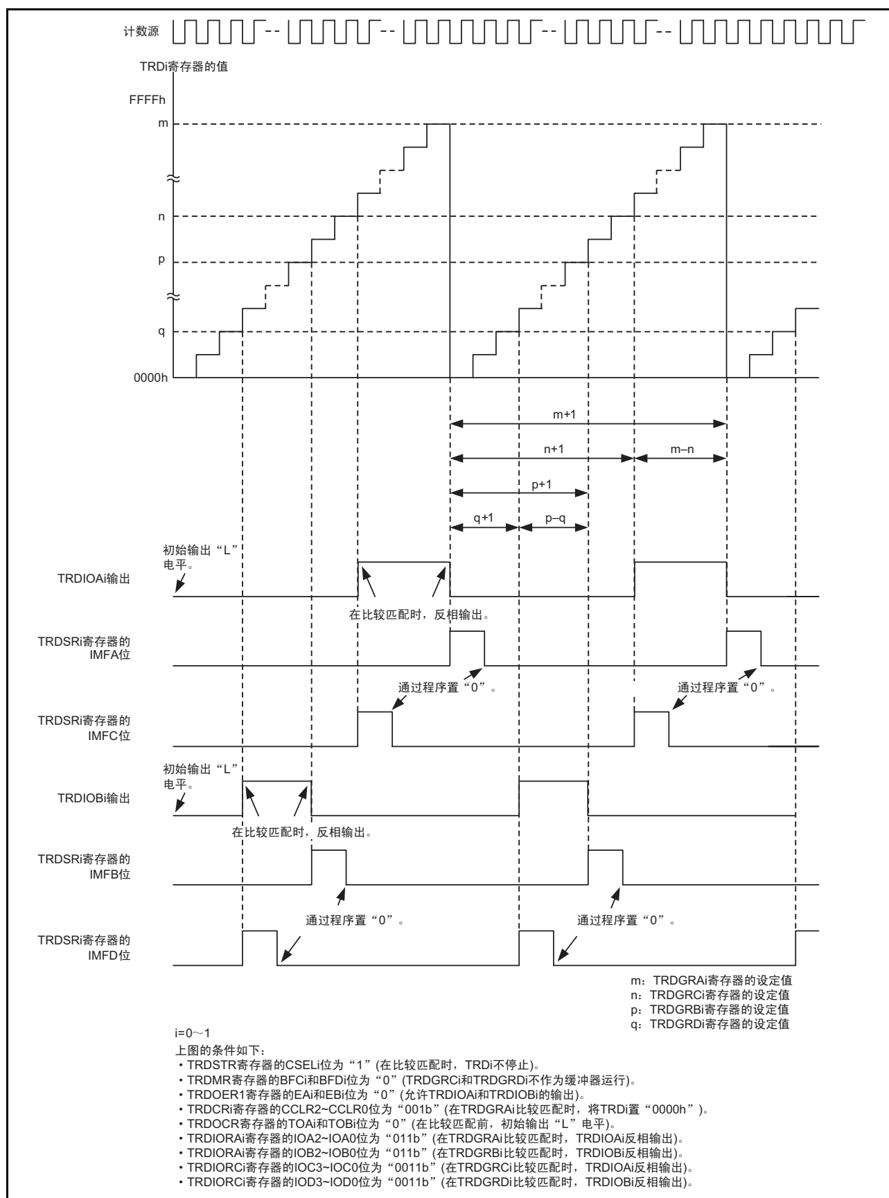
图 20.13 将 TRDGRGi 和 TRDGRDi 分别用于 TRDIOAi 引脚和 TRDIOBi 引脚的输出控制时的运行例子
