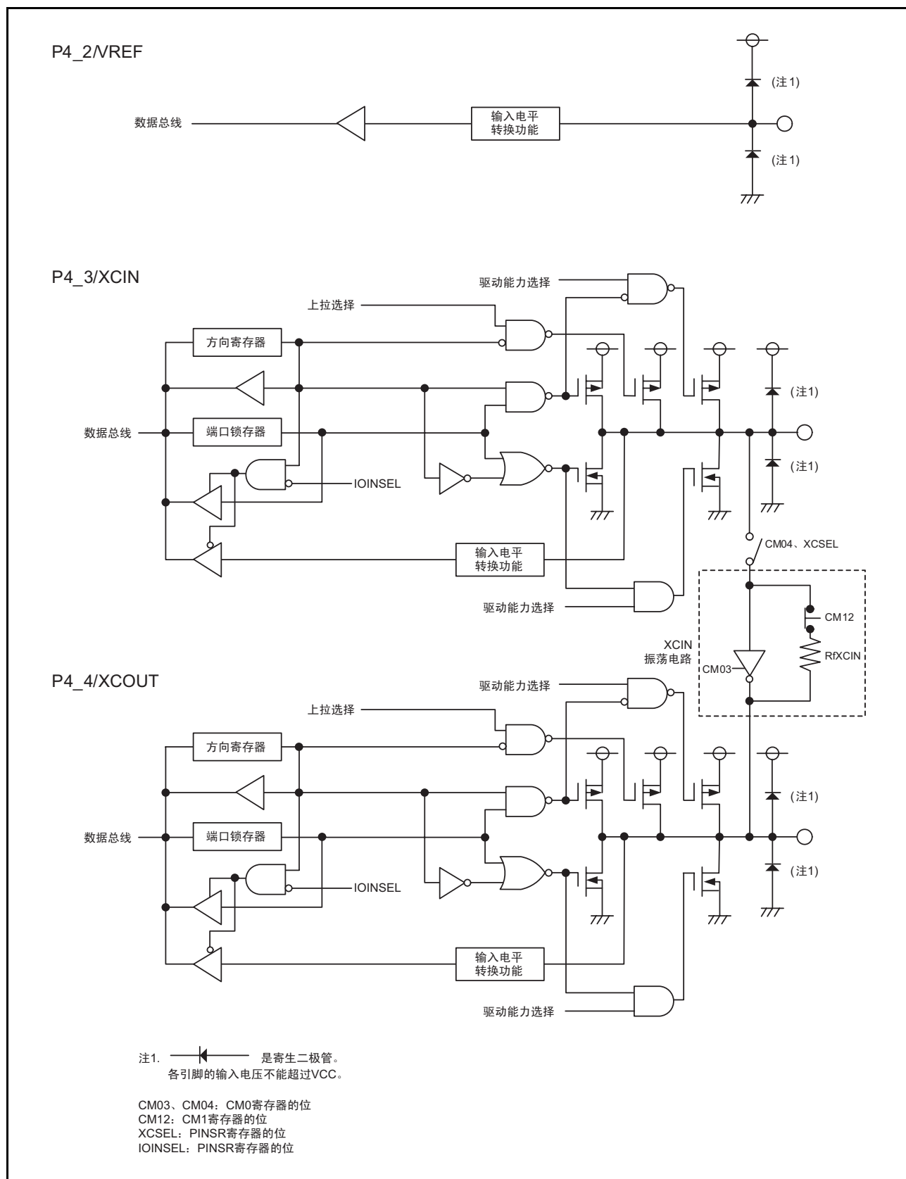
图 7.10 I/O 端口的结构 (10)
