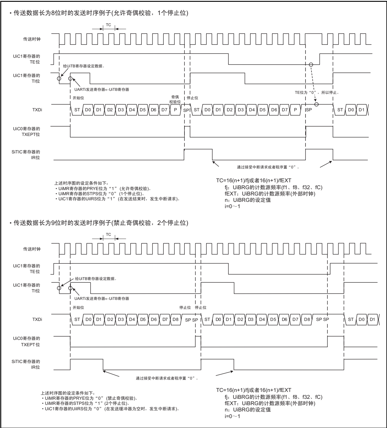
图 22.6 UART 模式的发送时序
