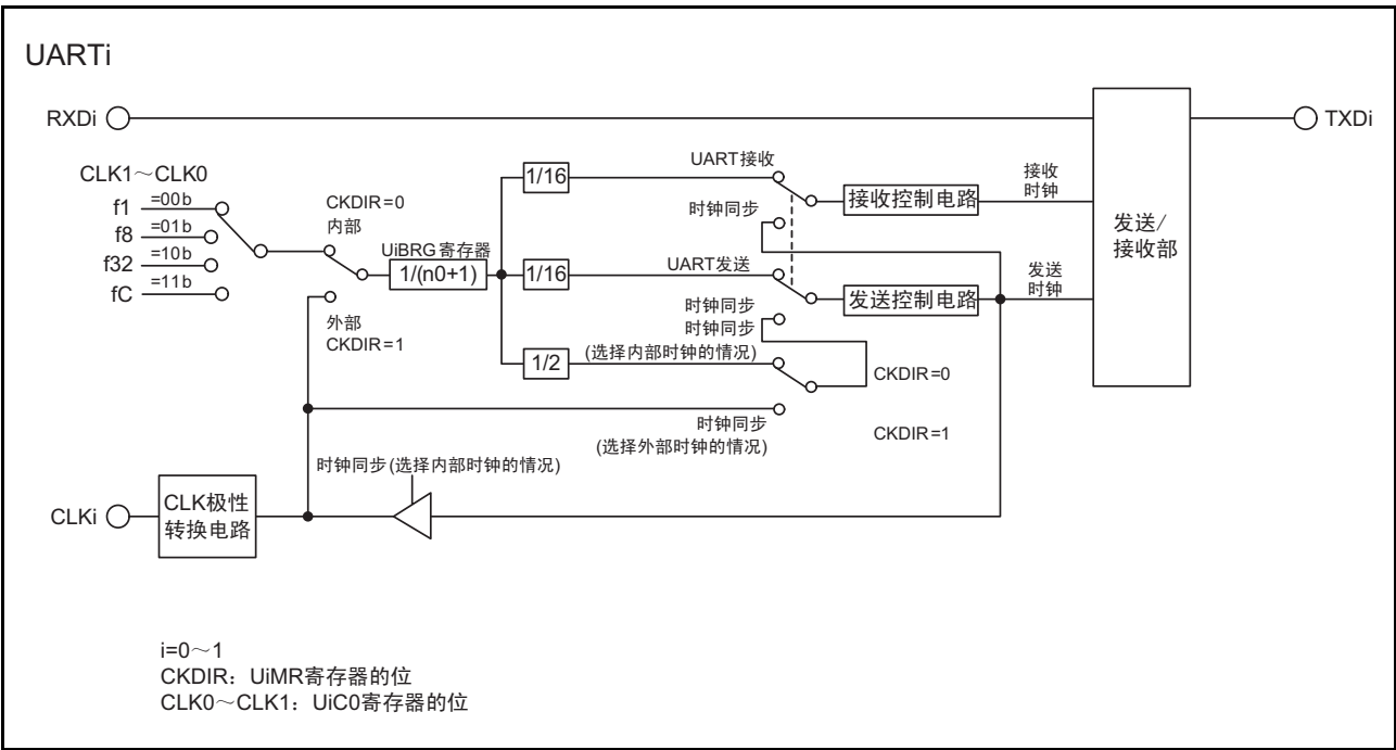
图 22.1 UARTi (i=0 ~ 1) 的框图
