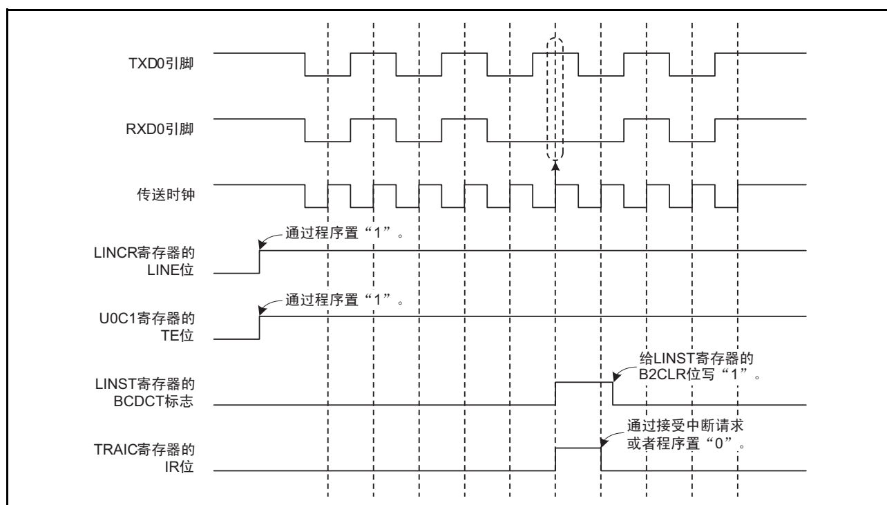
图 27.9 检测总线冲突时的运行例子
