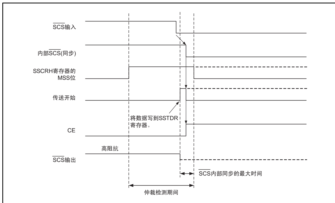
图 25.13 仲裁检查时序
