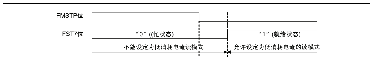
图 31.3 转移到低消耗电流读模式
