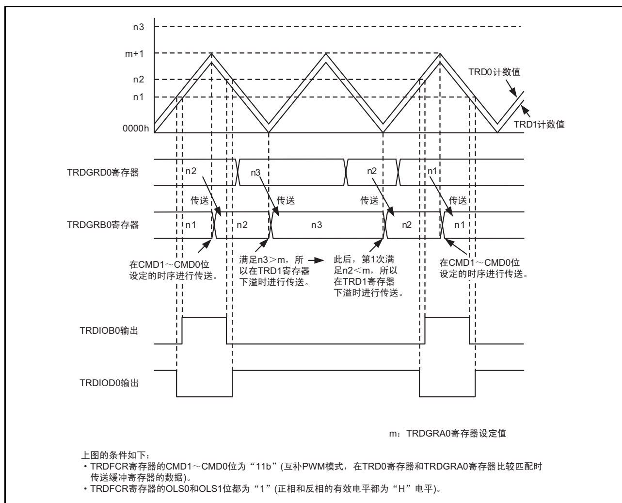
图 20.27 互补 PWM 模式中的缓冲寄存器的值 \geq TRDGRA0 寄存器的值时的运行例子
