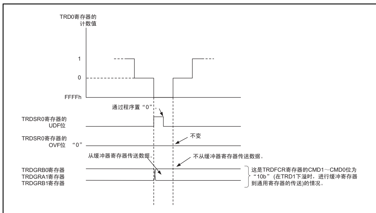
图 34.3 互补 PWM 模式中的 TRD1 发生下溢时的运行例子
