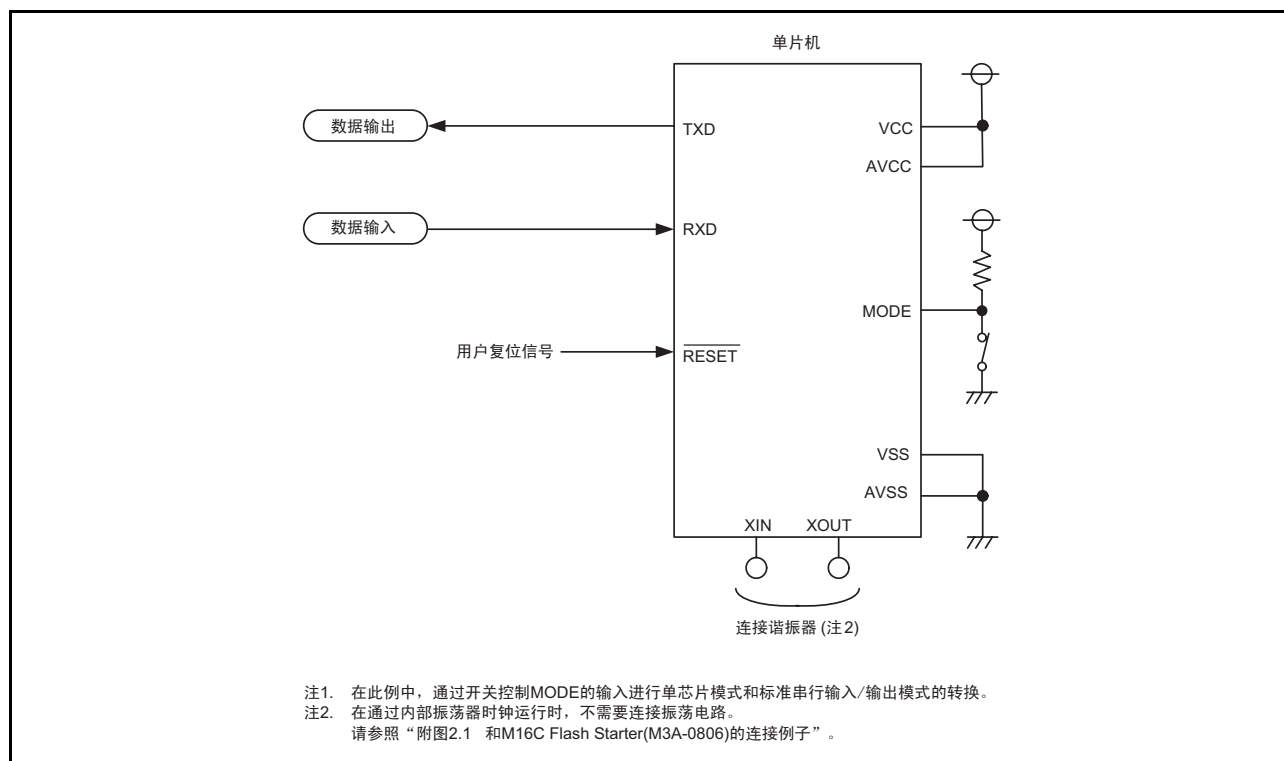
图 31.18 使用标准串行输入 / 输出模式 2 时的引脚处理例子
