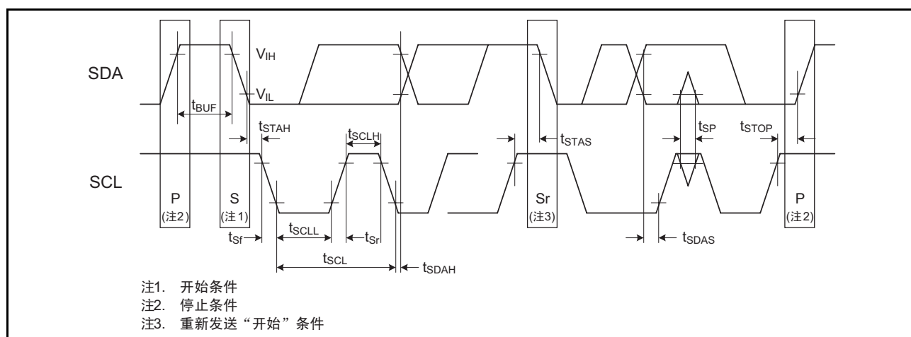
图 33.7 I 2 C 总线接口的输入 / 输出时序
