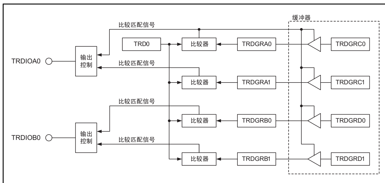
图 20.22 PWM3 模式的框图
