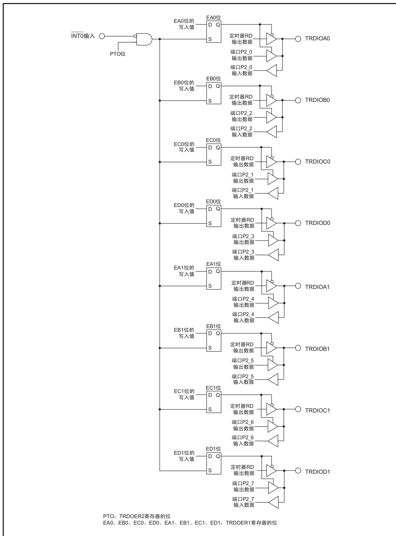
图 20.6 脉冲输出的强制截止
