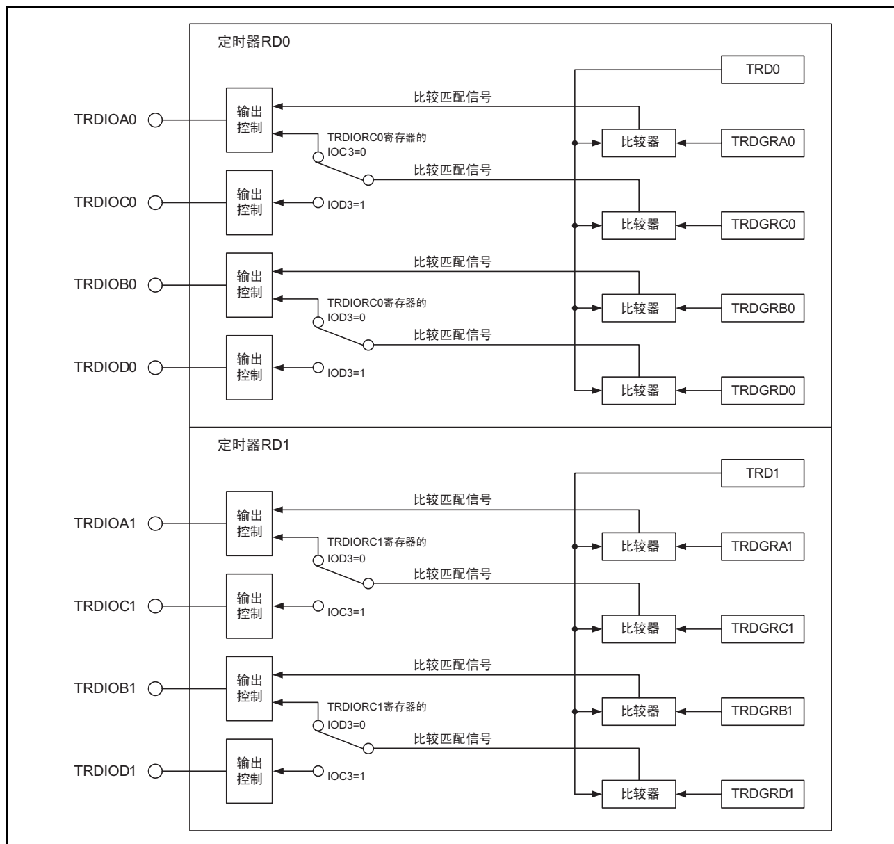
图 20.12 TRDGRCi 和 TRDGRDi 的输出引脚的变更
