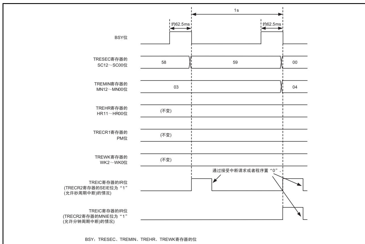
图 21.3 实时时钟模式的运行例子
