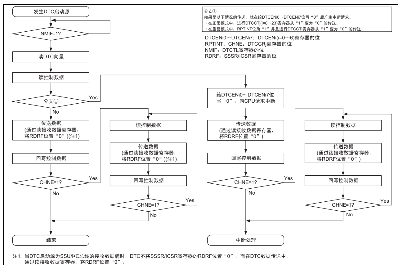
图 15.5 DTC 的内部运行流程图（DTC 启动源是 SSU/I²C 总线的接收数据满）
