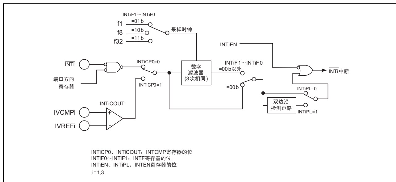
图 30.3 比较电路 Bi 数字滤波器的结构
