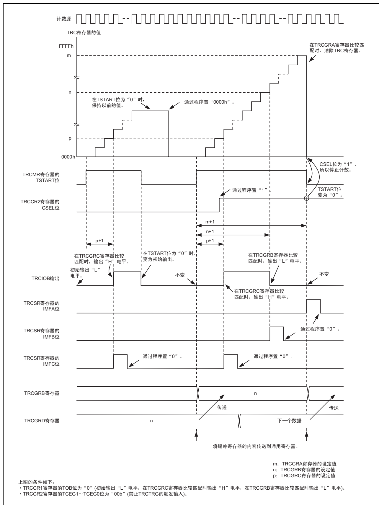
图 19.17 PWM2 模式的运行例子（禁止 TRCTRIG 触发输入）
