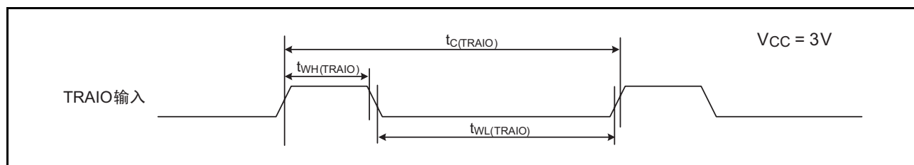
图 33.13 V_{CC}=3V 时的 TRAIO 输入时序
