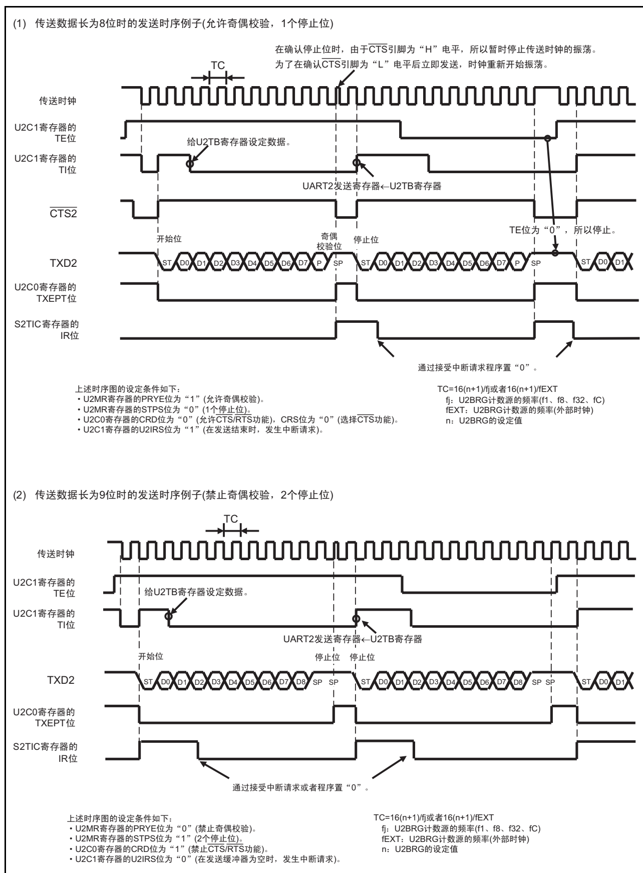
图 23.7 UART 模式的发送时序例子
