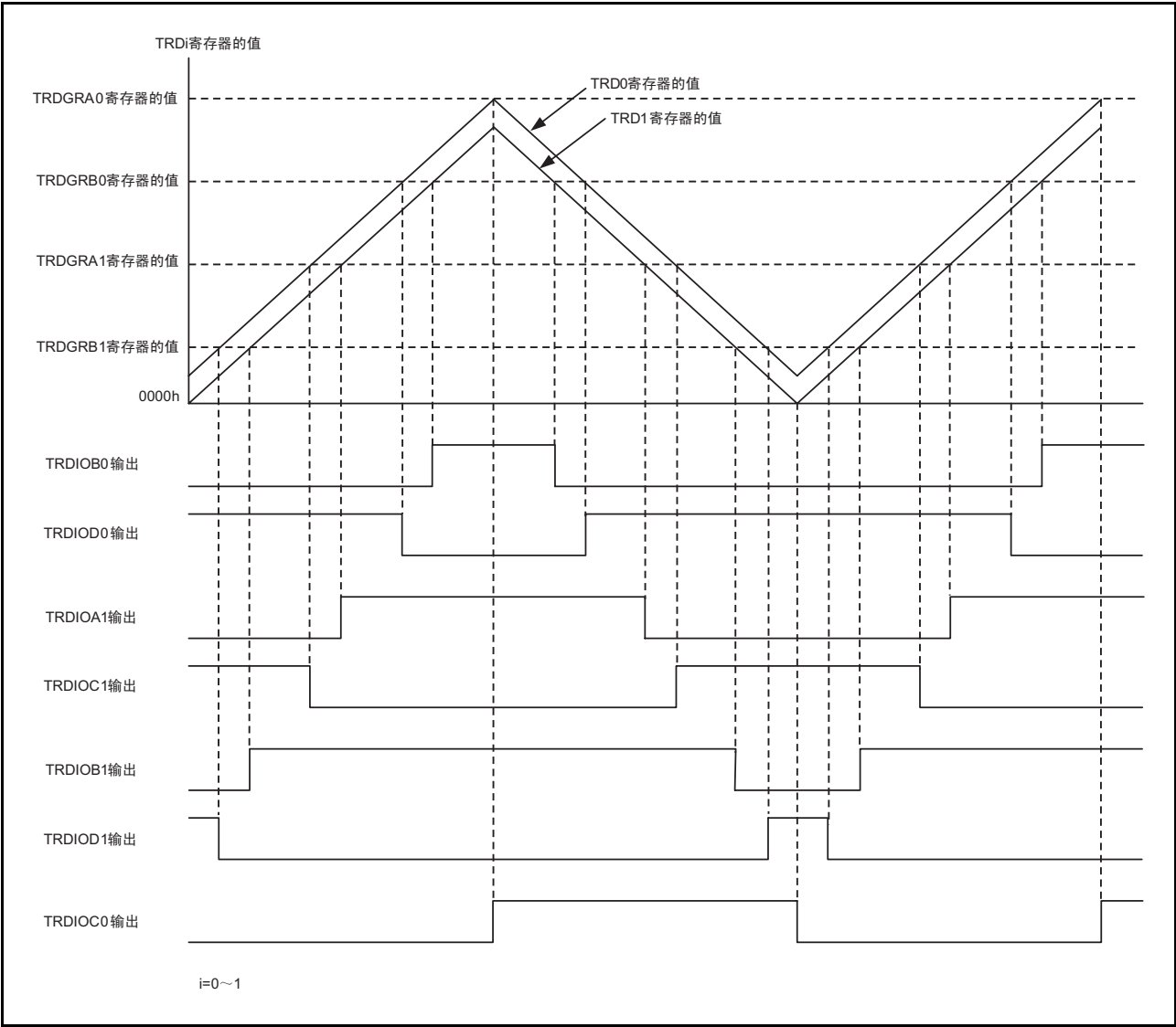
图 20.20 互补 PWM 模式的输出模型
