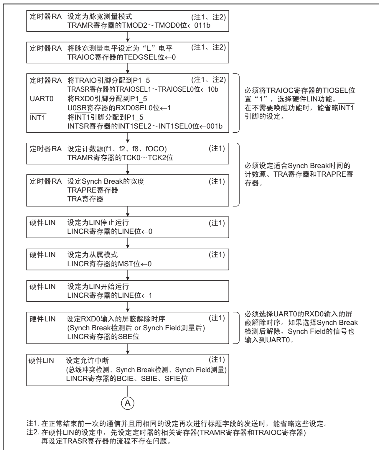
图 27.6 标题字段的接收流程图例子 (1)
