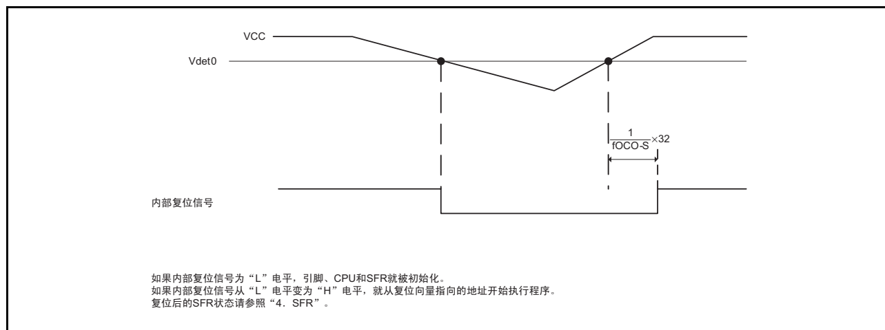
图 6.5 电压监视 0 复位的运行例子
