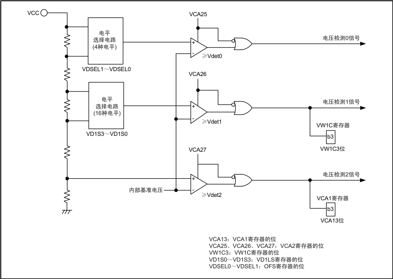
图 6.1 电压检测电路的框图
