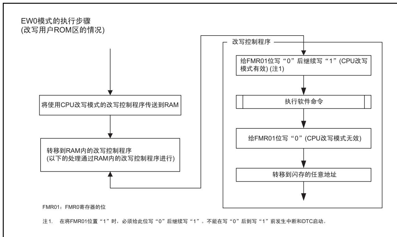
图 31.5 EW0 模式的设定和解除方法
