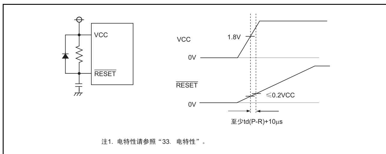
图 5.4 硬件复位的电路例子和运行
