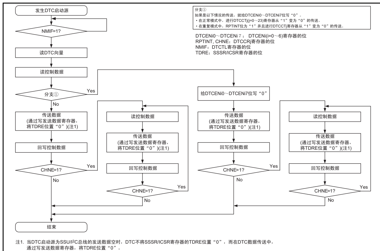
图 15.6 DTC 的内部运行流程图（DTC 启动源是 SSU/I²C 总线的发送数据空）
