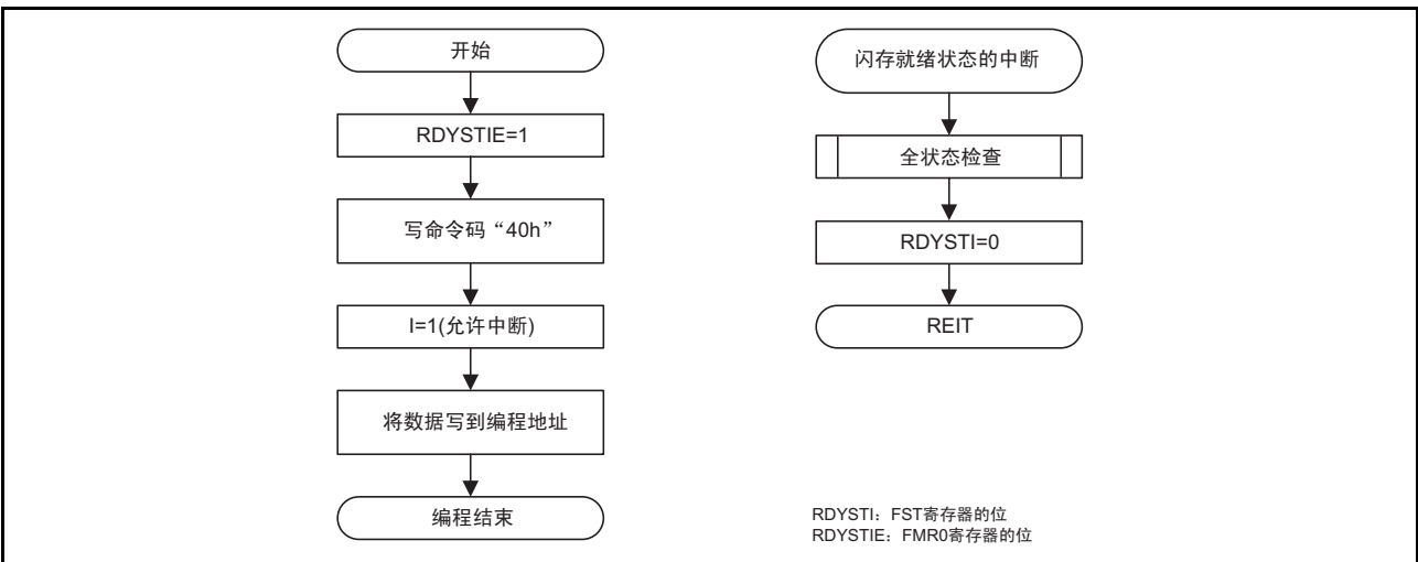
图 31.10 编程的流程图（允许闪存就绪状态的中断）
