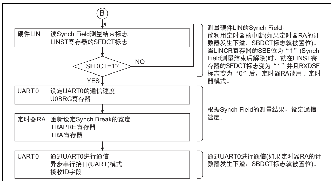
图 27.8 标题字段的接收流程图例子 (3)
