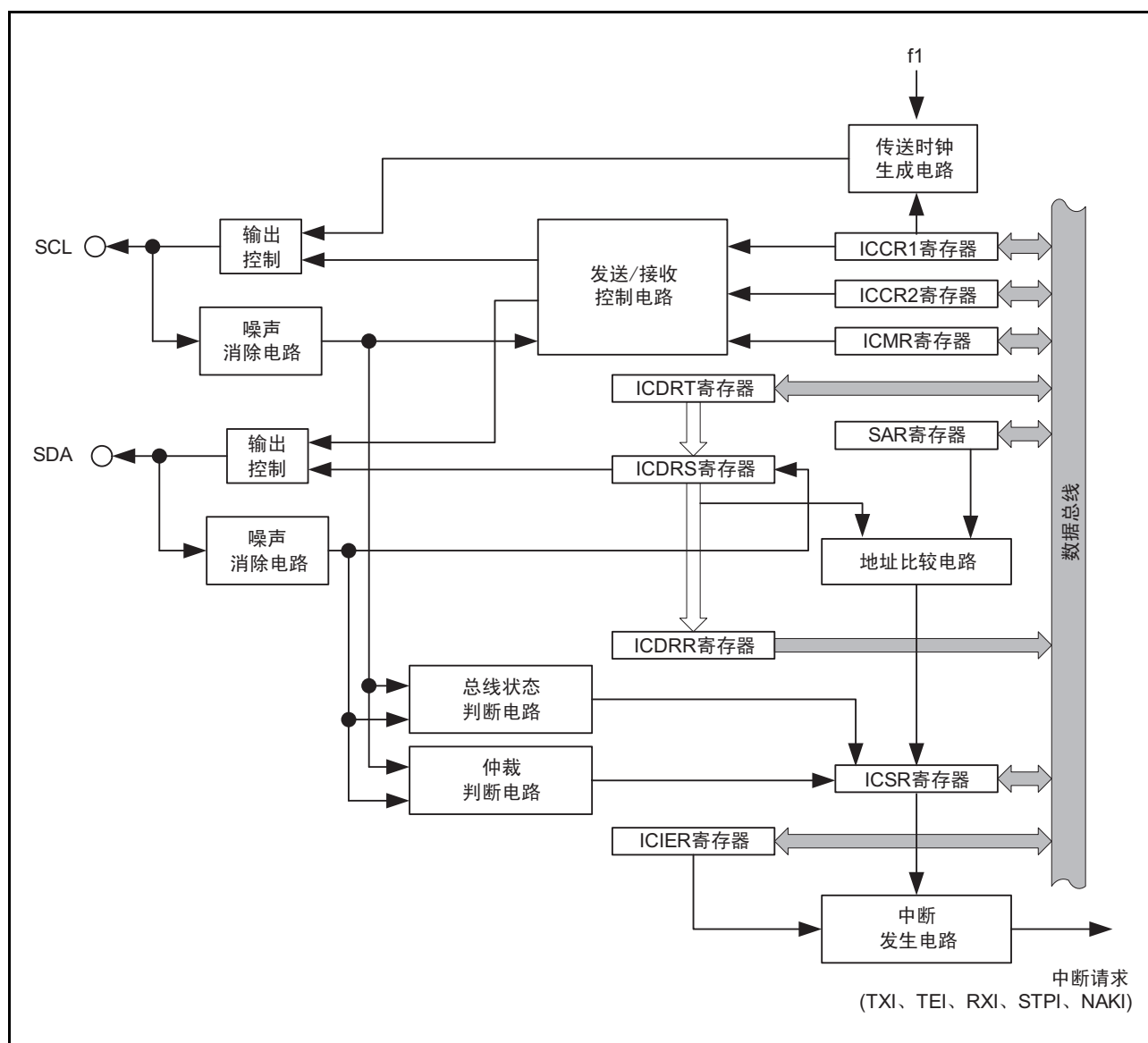
图 26.1 I 2 C 总线接口的框图
