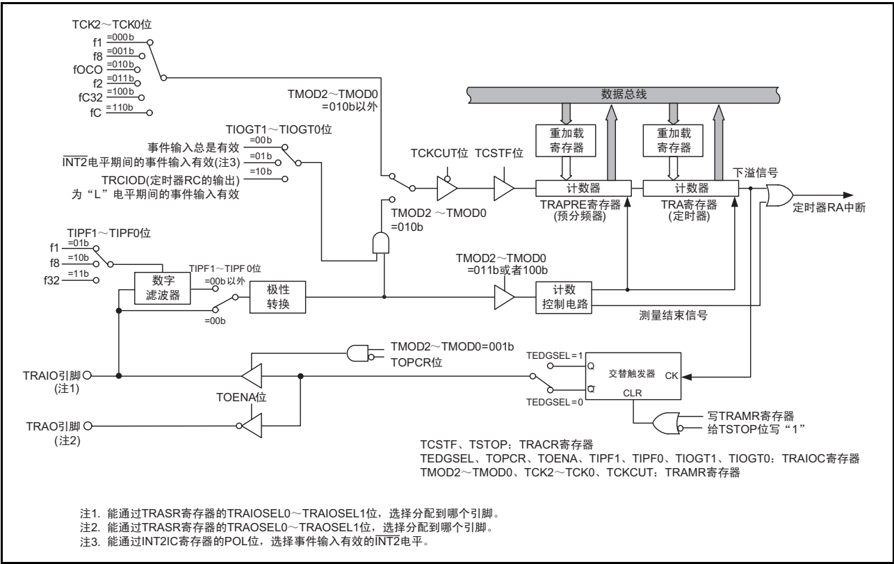
图 17.1 定时器 RA 的框图
