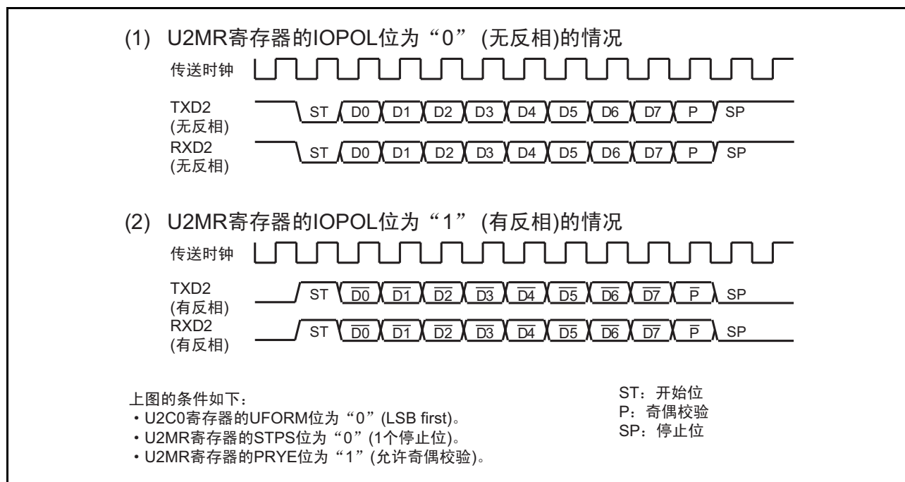
图 23.11 TXD 和 RXD 输入 / 输出极性的转换
