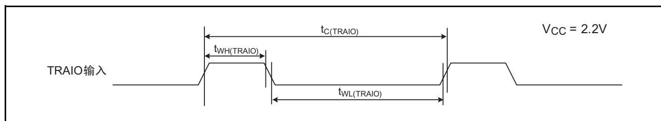
图 33.17 V_{CC}=2.2V 时的 TRAIO 输入时序
