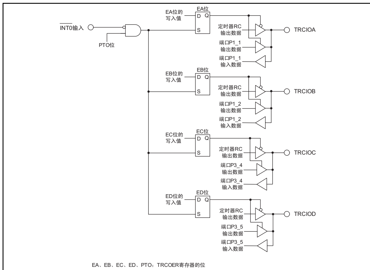
图 19.6 脉冲输出的强制截止
