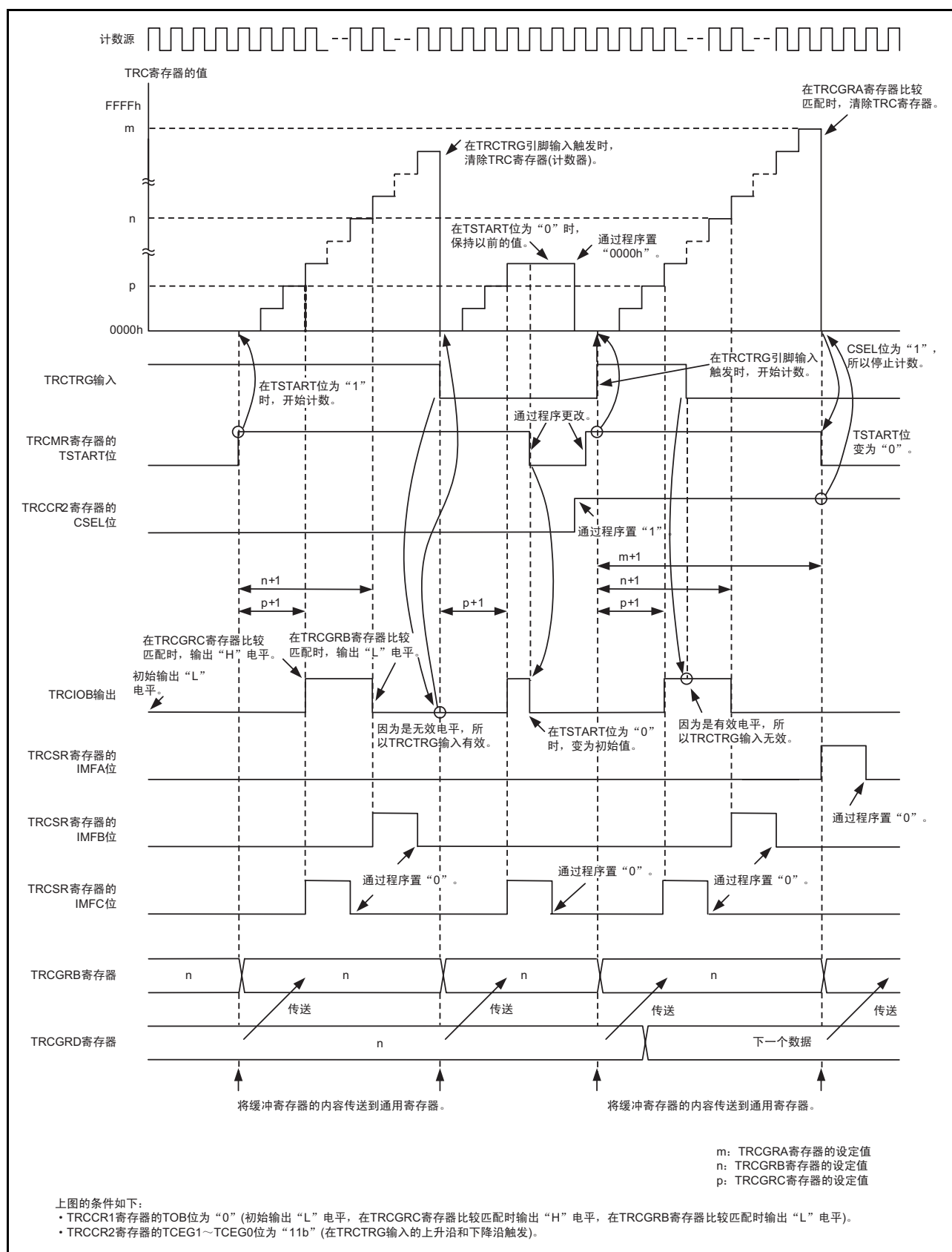
图 19.18 PWM2 模式的运行例子（允许 TRCTRIG 触发输入）
