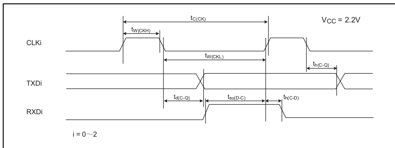
图 33.18 V_{CC}=2.2V 时的串行接口时序
