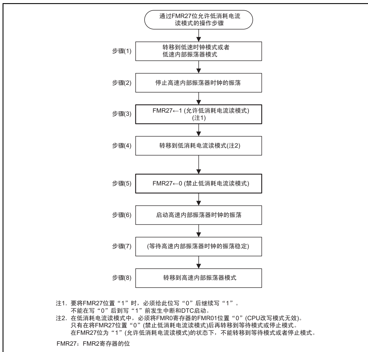
图 32.3 低消耗电流读模式的操作步骤例子
