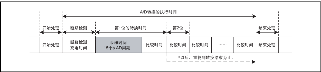
图 28.2 A/D 转换时序图
