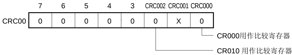
(b) 16 位定时器输出控制寄存器 00 (TOC00)
