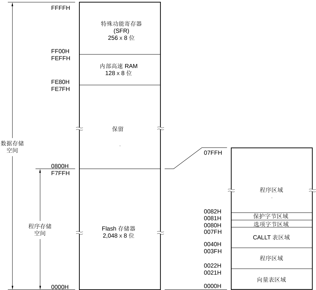
图 3-1. 存储空间映射图 (μPD78F9221)
