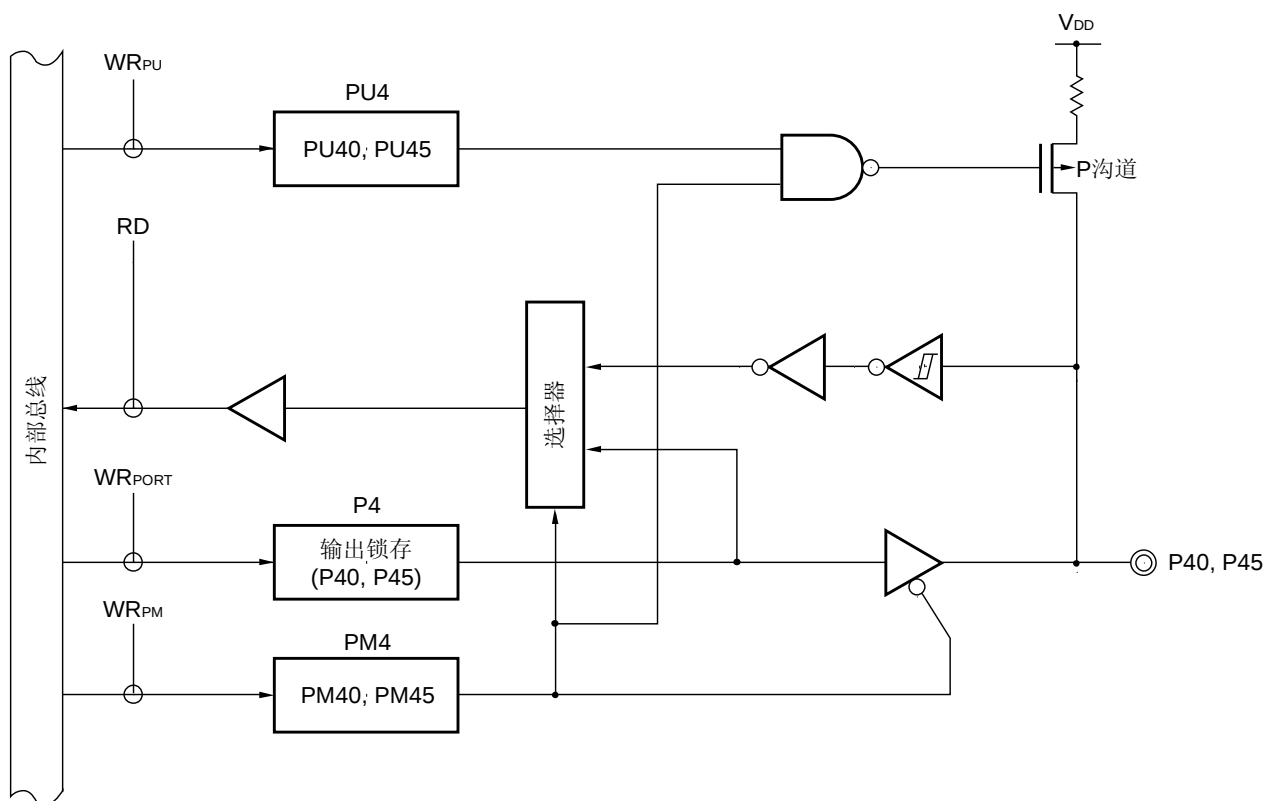
图 4-6 P40 和 P45 的框图
