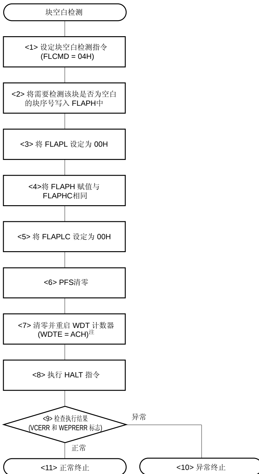
图 18-21. 在自编程模式下空白块校验操作流程
