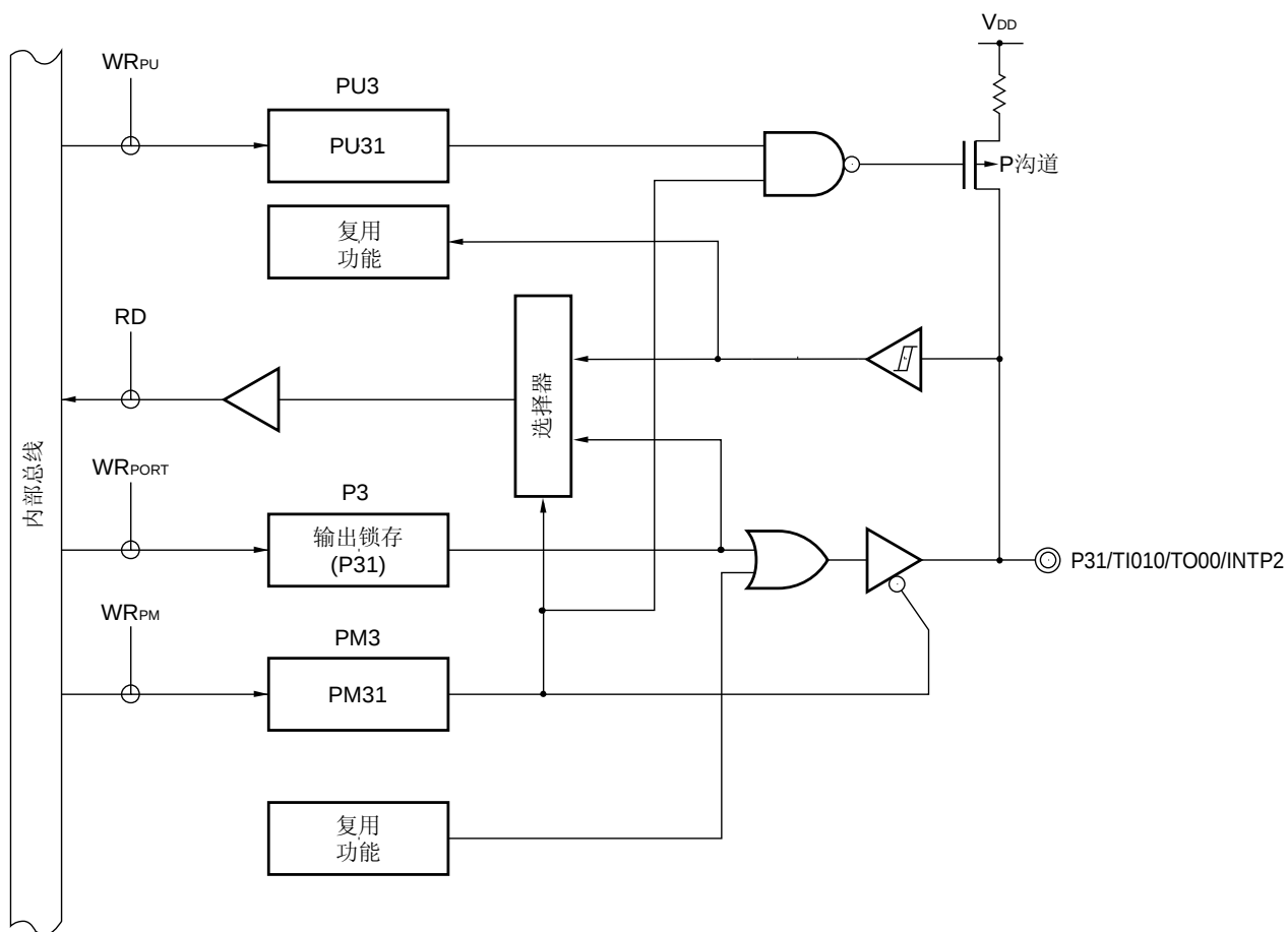
图 4-4 P31 的框图
