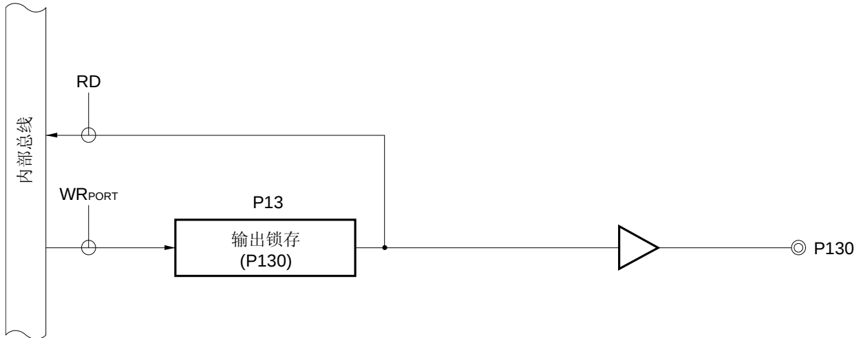
图 4-12 P130 的框图
