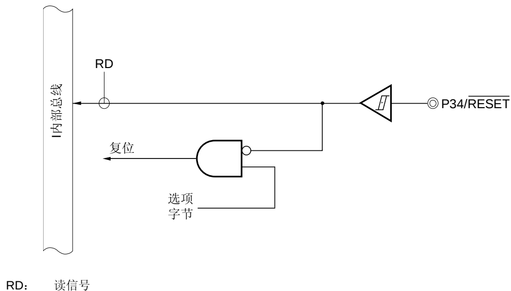
图 4-5 P34 的框图
