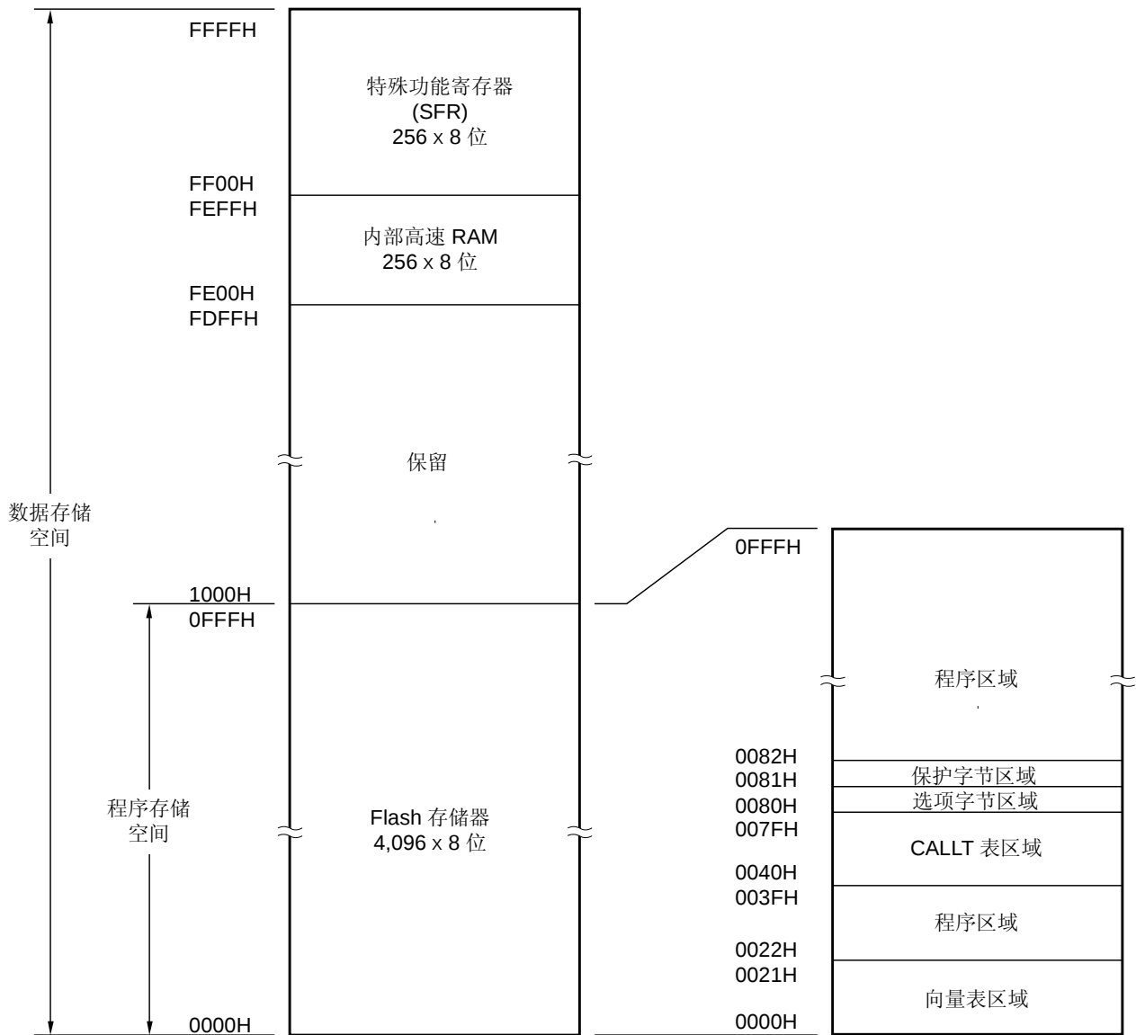
图 3-2. 存储空间映射图 (μPD78F9222)
