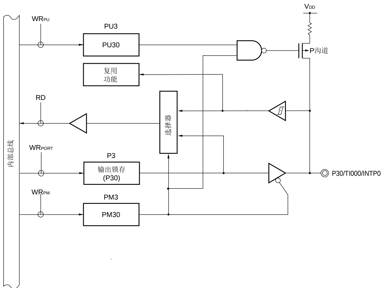
图 4-3 P30 的框图
