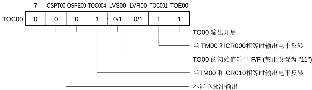
(c) 预分频模式寄存器 00 (PRM00)
