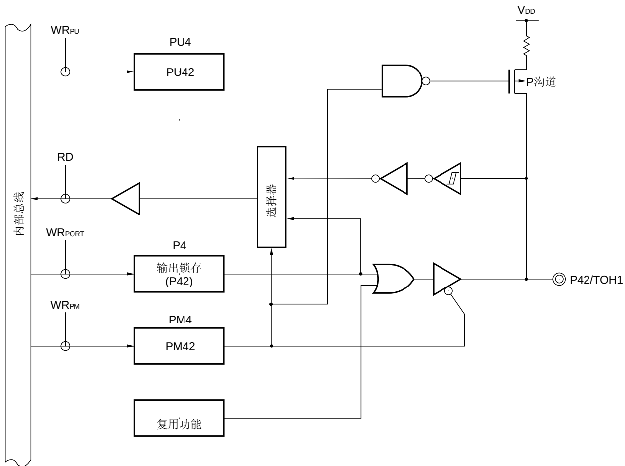
图 4-8 P42 的框图
