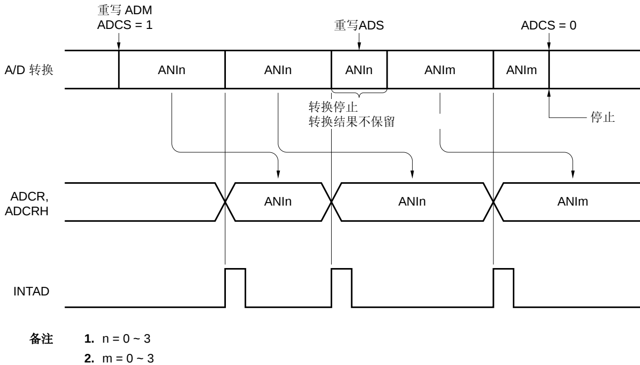
图 10-12 A/D 转换操作
