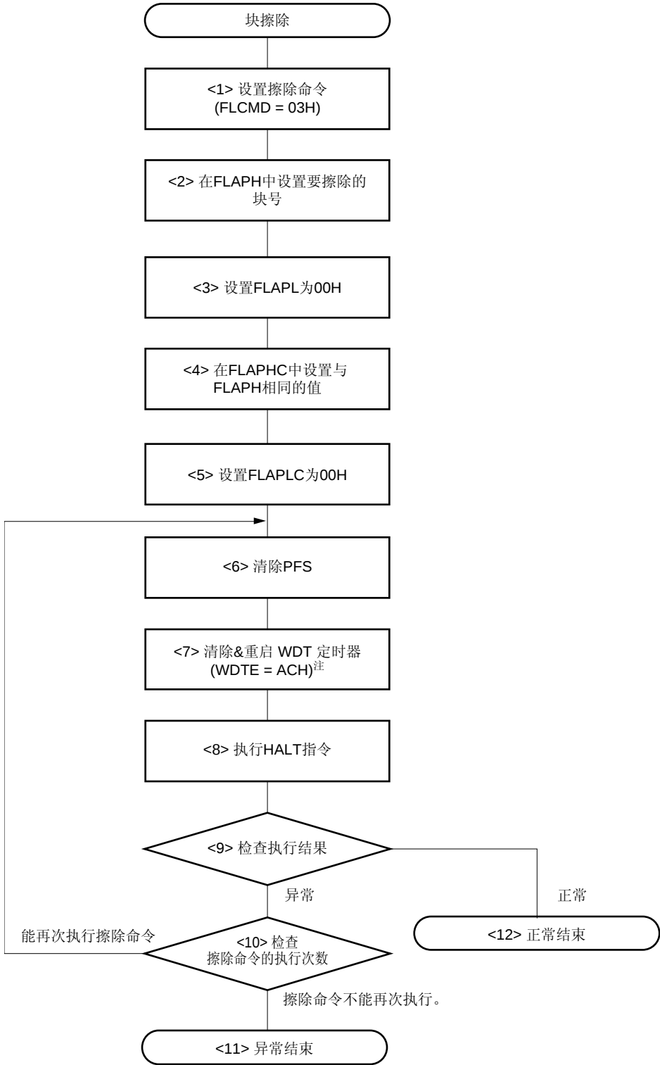
图 18-20. 自编程模式下块擦除操作流程
