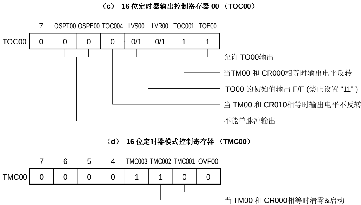
图 6-27. 方波输出模式下控制寄存器的设置 (2/2)
