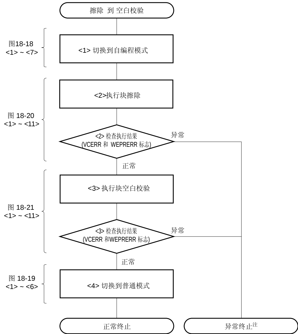
图 18-25 最短命令执行时间的操作流程（从擦除到空白检验）
