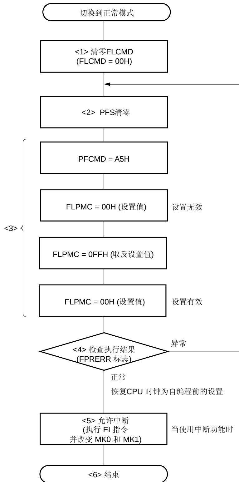
图 18-19. 切换到正常模式示例
