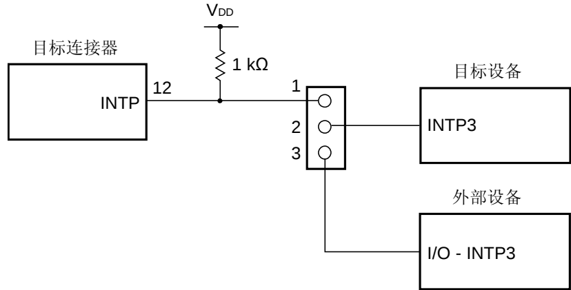
图19-4. QB-MINI2用来调试且INTP3引脚的调试只能通过实际设备来执行时的线路连接
