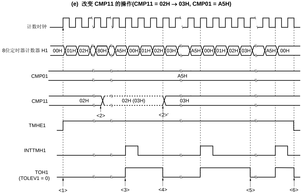
图 8-9. PWM 输出模式下的时序操作 (4/4)
