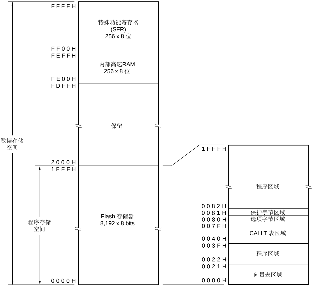
图 3-3. 存储空间映射图(μPD78F9224)
