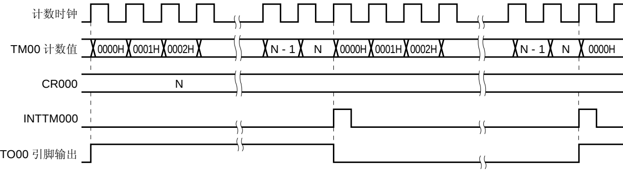
图 6-28. 方波输出操作时序
