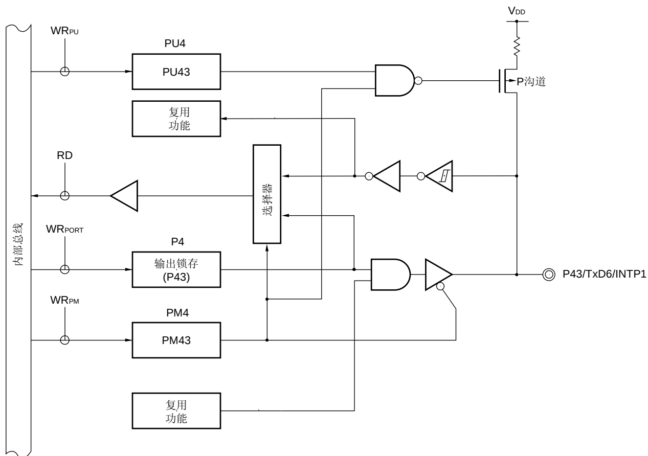
图 4-9 P43 的框图
