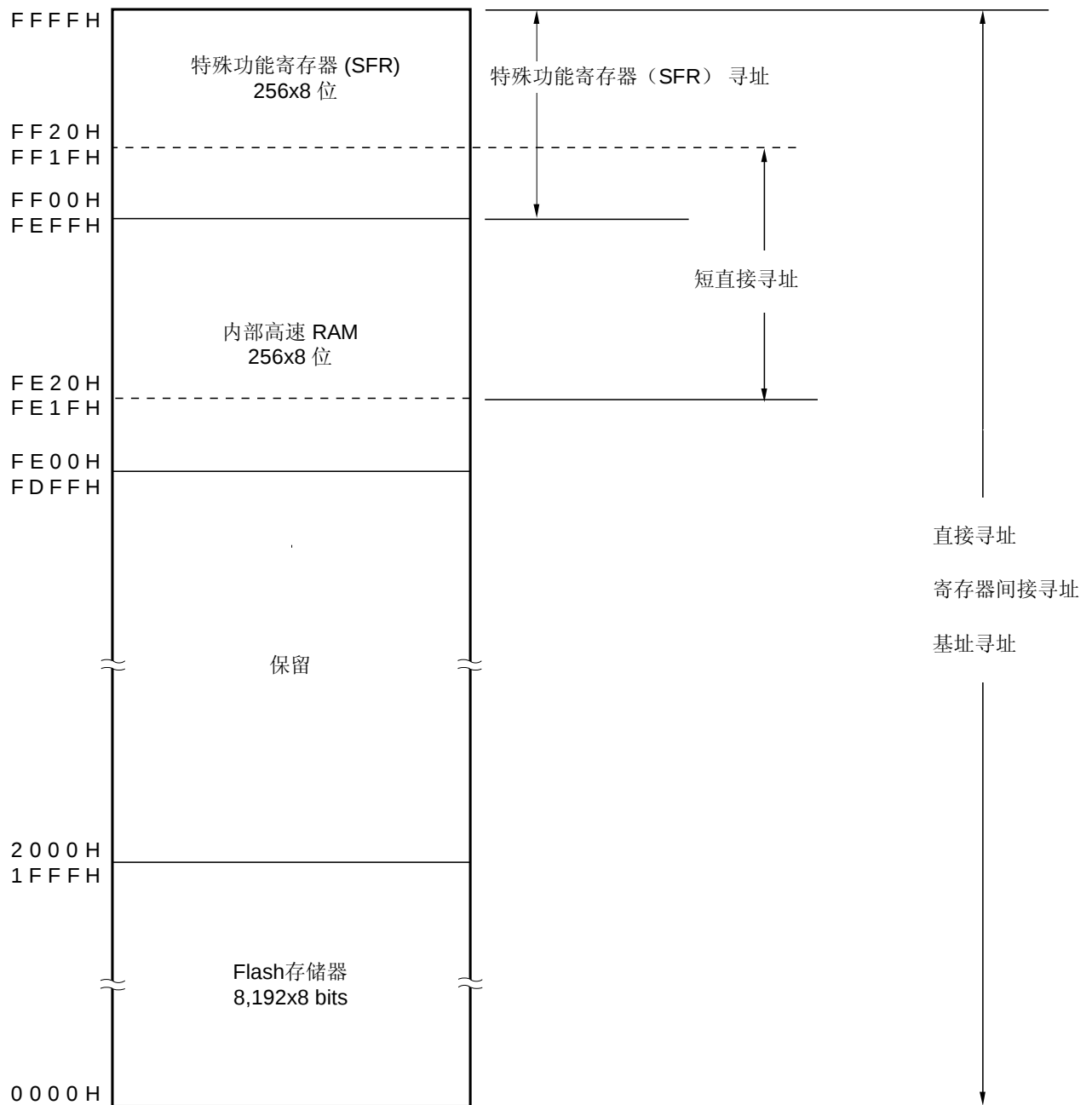
图 3-6. 数据存储寻址 (μPD78F9224)
