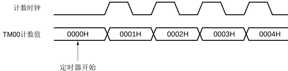
图 6-36. 16 位定时器计数器 00 (TM00) 的启动时序
