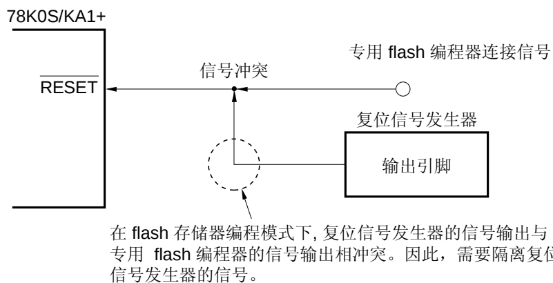
图 18-6. 信号冲突 (RESET 引脚)
