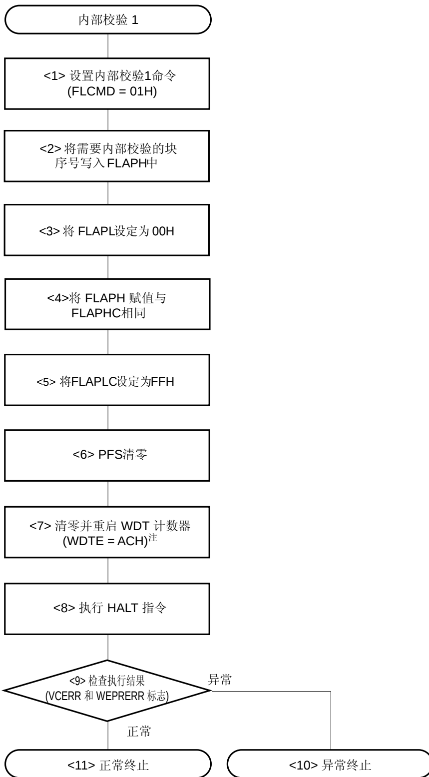
图 18-23. 自编程模式下内部校验 1 流程
