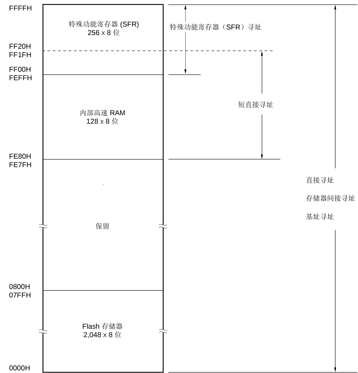
图 3-4. 数据存储器寻址（ \mu PD78F9221）
