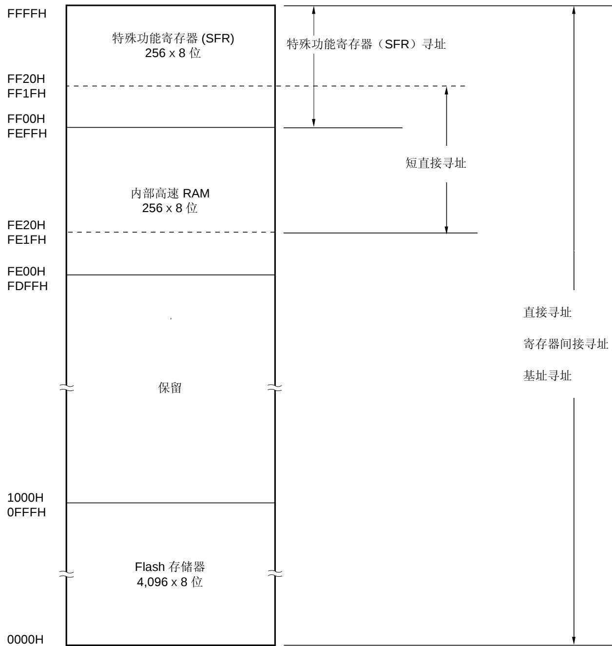
图 3-5. 数据存储器寻址 (μPD78F9222)
